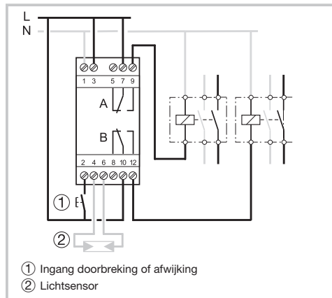
Afbeelding 2: aansluitingsschema EGN200 (2 uitgangen)
