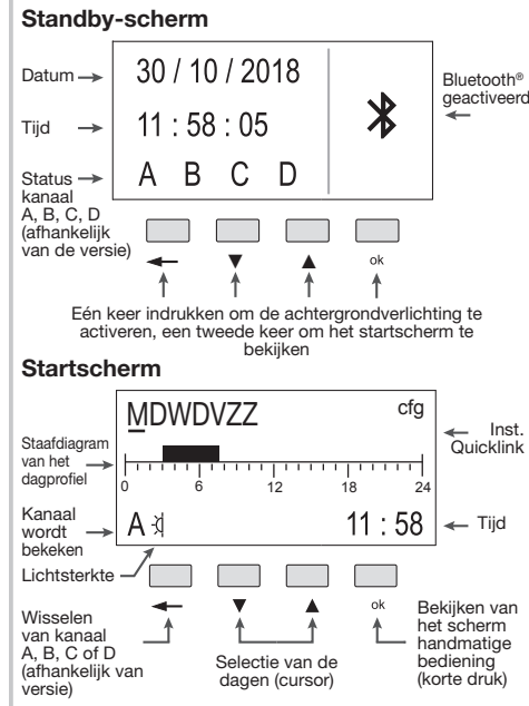
Afbeelding 1: weergave van het standby- en startscherm
