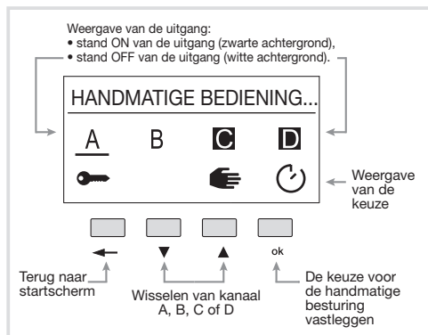
Afbeelding 4: weergave van het scherm voor handmatige besturing.
