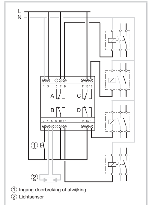
Afbeelding 3: aansluitingsschema EGN400 (4 uitgangen)
