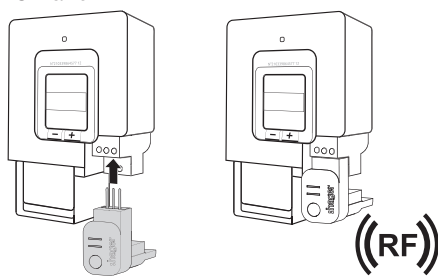
Bild 2: Anschluss der CHP-Funktionen
