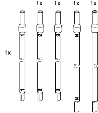
Y883F Abgangskabelbaum 5-polig
