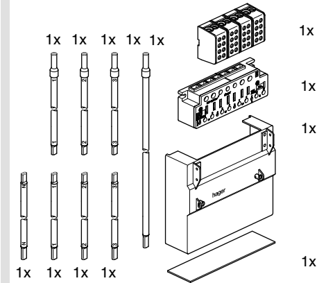
ZY101 Bestückungspaket 4-polig
