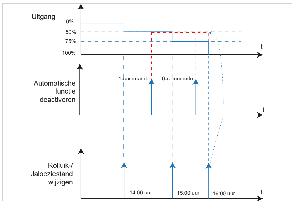
Afbeelding 57: Signaal-tijdschema Automatische functie deactiveren
