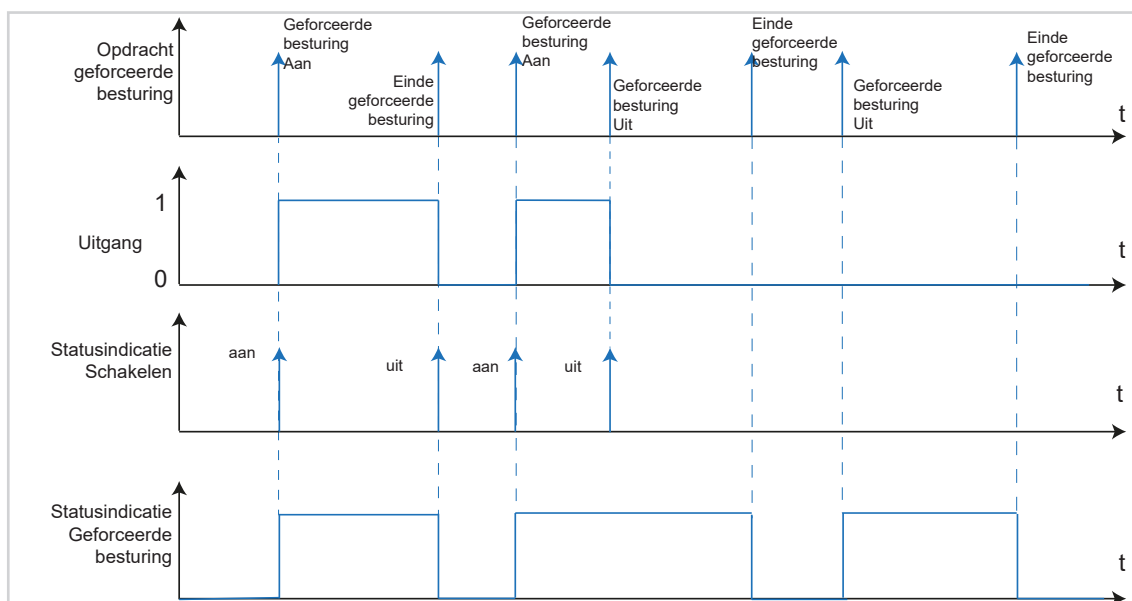
Afbeelding 26: Signaal-tijd diagram Geforceerde besturing
