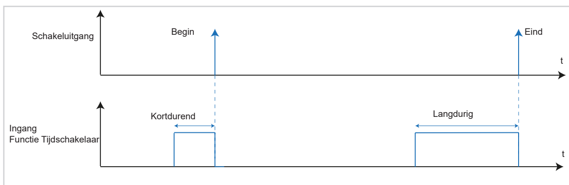
Afbeelding 23: Signaal-tijdschema Tijdschakelaar
