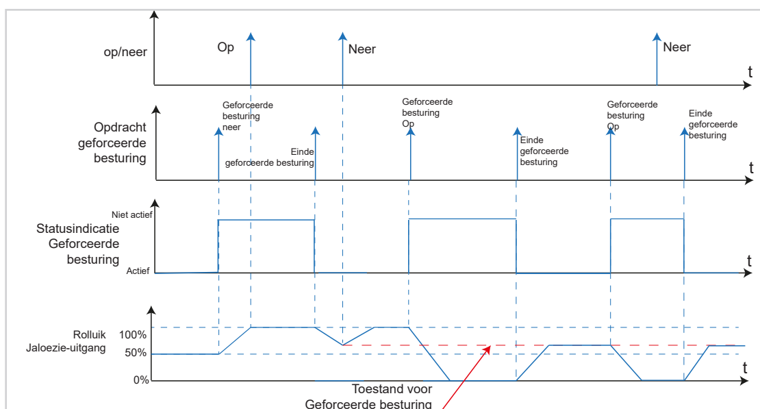
Afbeelding 55: Signaal-tijd diagram Geforceerde besturing rolluik/jaloezie
