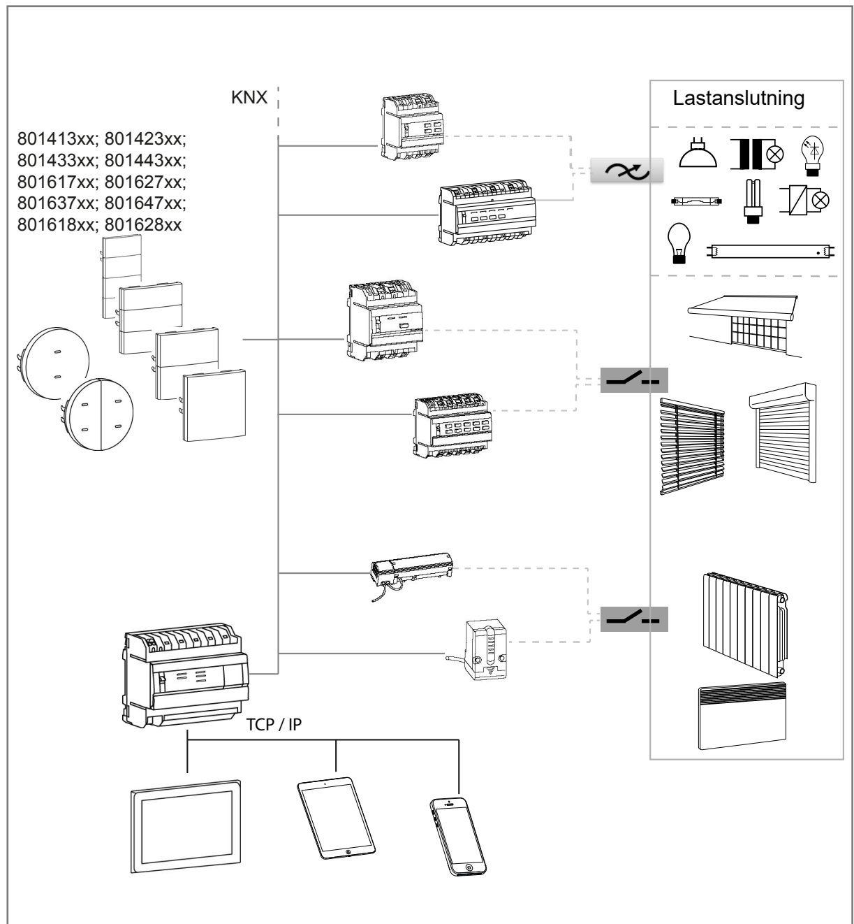
Bild 1: Enhetsöversikt
