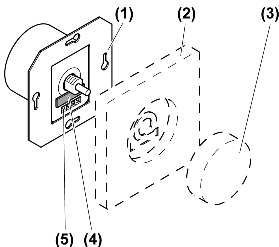
Bild 1: Enhetens konstruktion
