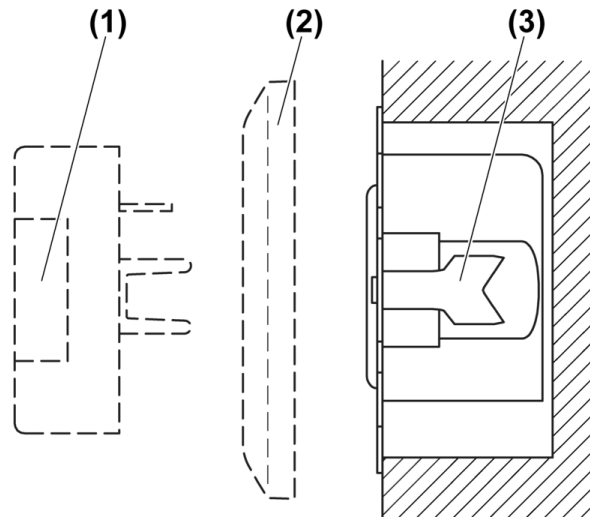
Afbeelding 1: Constructie apparaat
