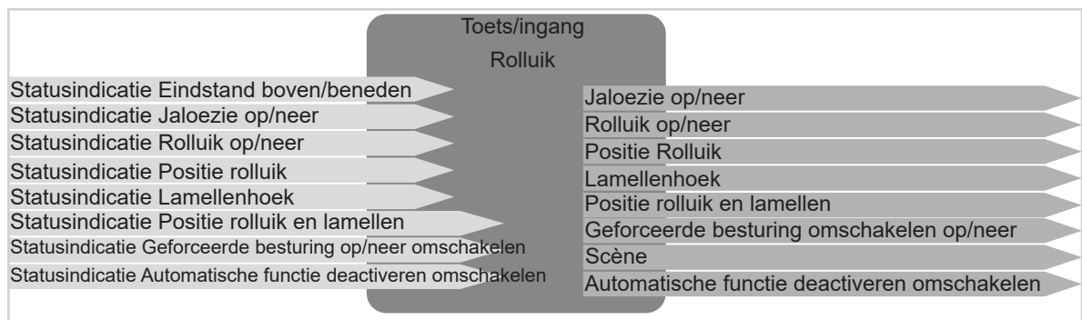
Afbeelding 6: In-/Uitgangssignalen functie rolluik
