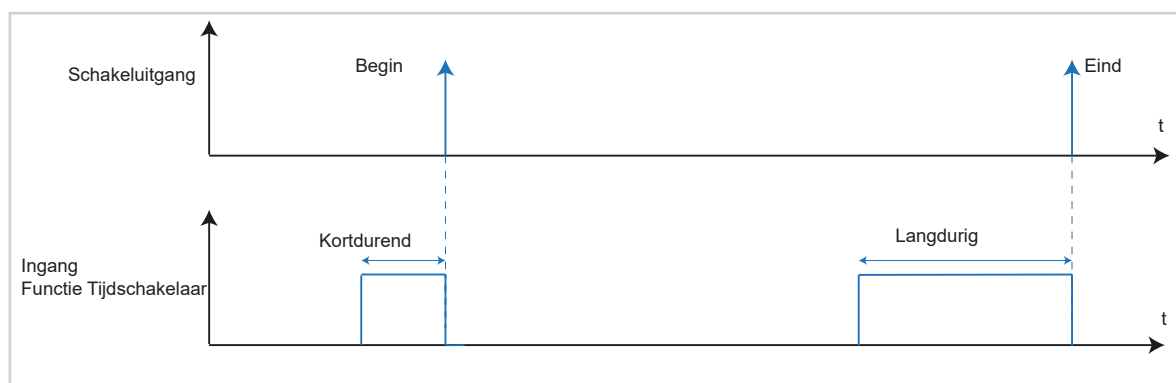
Afbeelding 21: Signaal-tijdschema Tijdschakelaar
