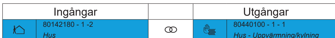
Bild 60: Sammankoppling funktionen Standby
