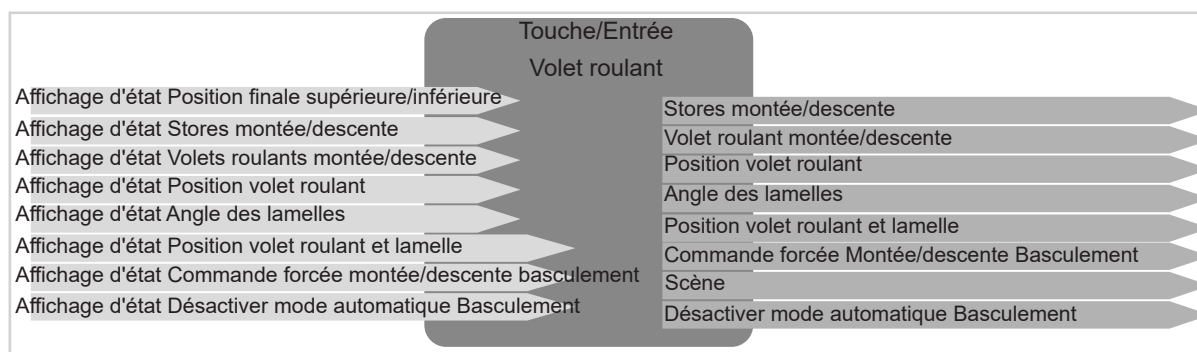
Image 6: Signaux d'entrée / de sortie Fonction Volet roulant
