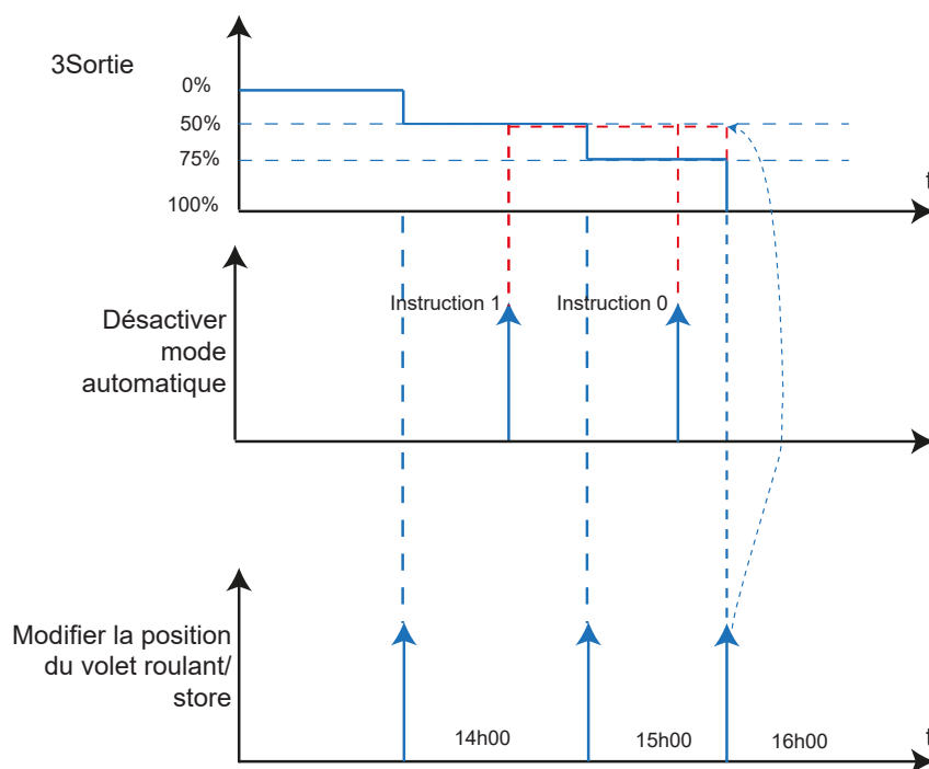
Image 55: Diagramme signal-temps Désactiver mode automatique
