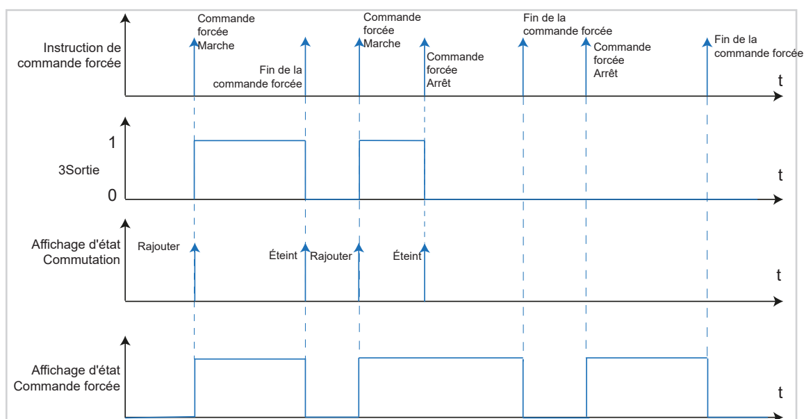
Image 24: Diagramme signal-temps Commande forcée
