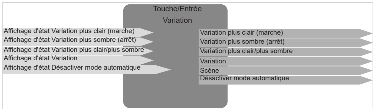
Image 5: Signaux d'entrée / de sortie Fonction Variation
