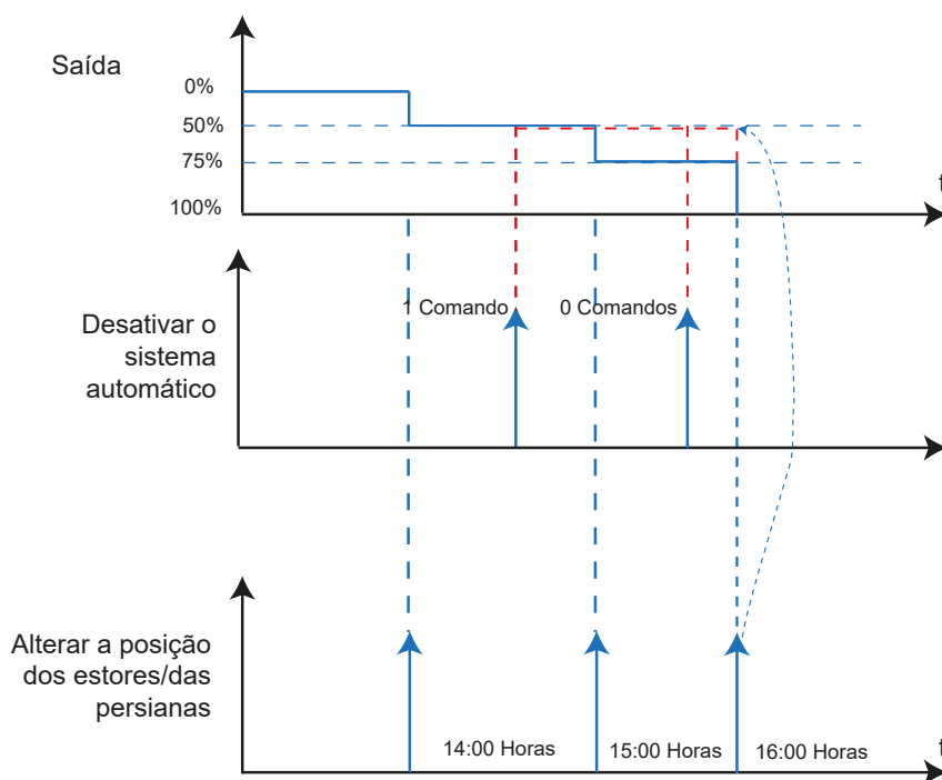
Figura 55: Diagrama de sinal e tempo Desativar o sistema automático
