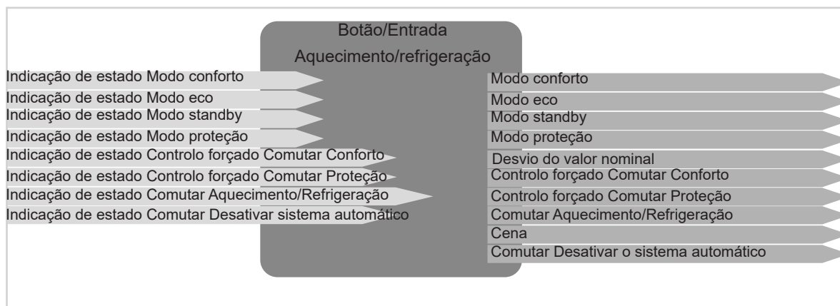
Figura 7: Sinais de entrada/saída Função aquecimento/refrigeração
