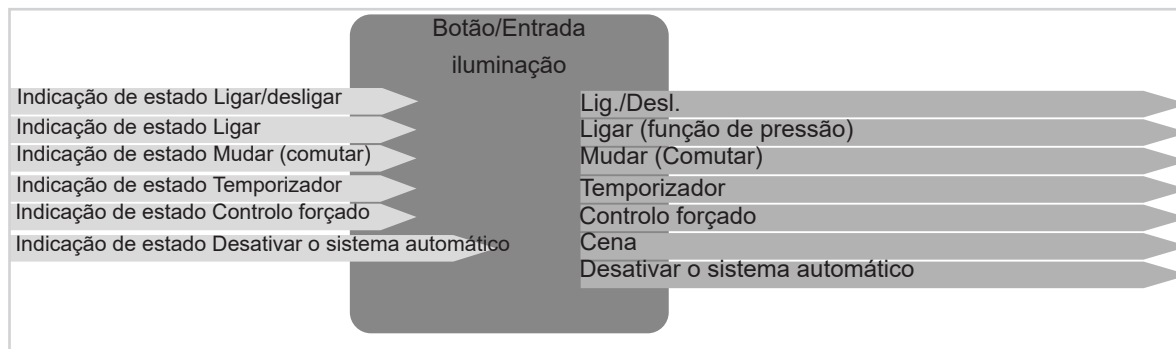
Figura 4: Sinais de entrada/saída Função iluminação
