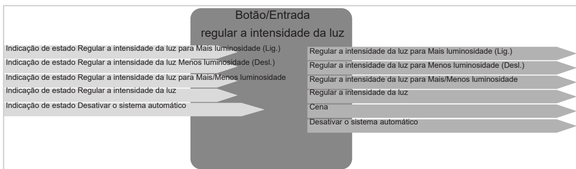
Figura 5: Sinais de entrada/saída Função de regulação da intensidade da luz
