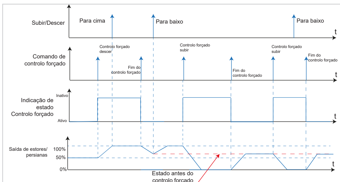
Figura 53: Diagrama de sinal e tempo Controlo forçado estore/persiana
