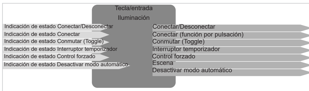
Figura 4: Señales de entrada/salida Función Iluminación
