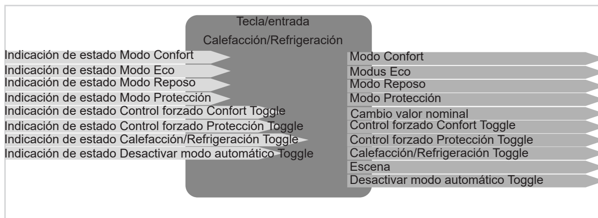
Figura 7: Señales de entrada/salida Función Calefacción/Refrigeración
