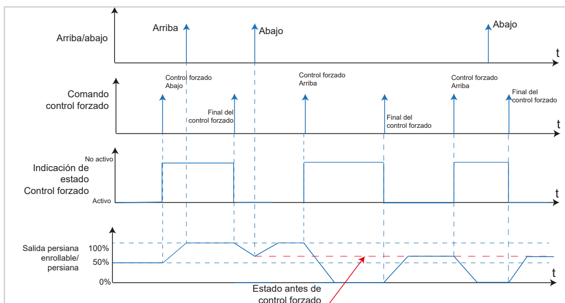
Figura 53: Gráfico señal-tiempo de Control forzado Persiana enrollable/Persiana
