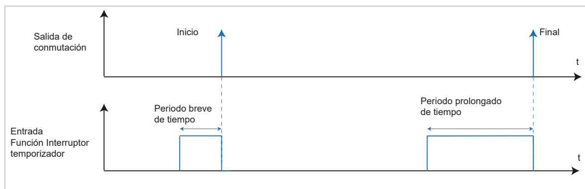
Figura 21: Gráfico señal-tiempo interruptor temporizador
