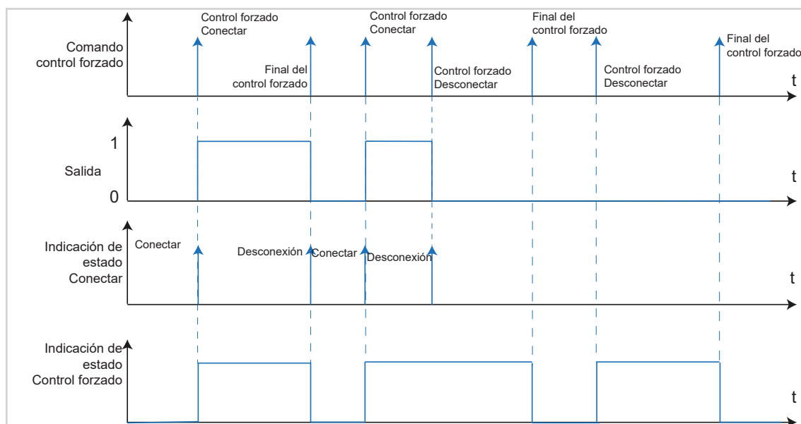
Figura 24: Gráfico señal-tiempo de control forzado
