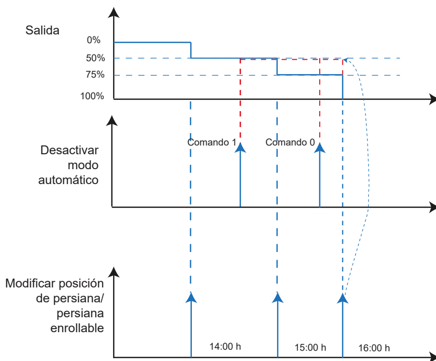
Figura 55: Gráfico señal-tiempo Desactivar modo automático
