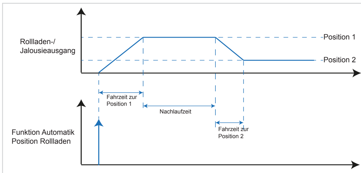
Bild 53: Signal-Zeit-Diagramm Automatik Position Rollladen
