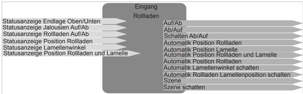
Bild 4: Ein-/Ausgangssignale Funktion Rollladen
