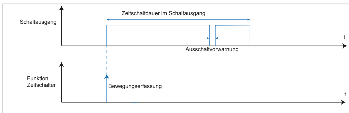
Bild 11: Signal-Zeit-Diagramm Zeitschalter
