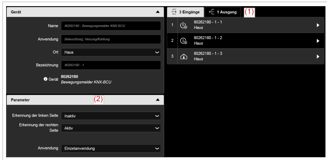
Bild 6: Geräteinformation
