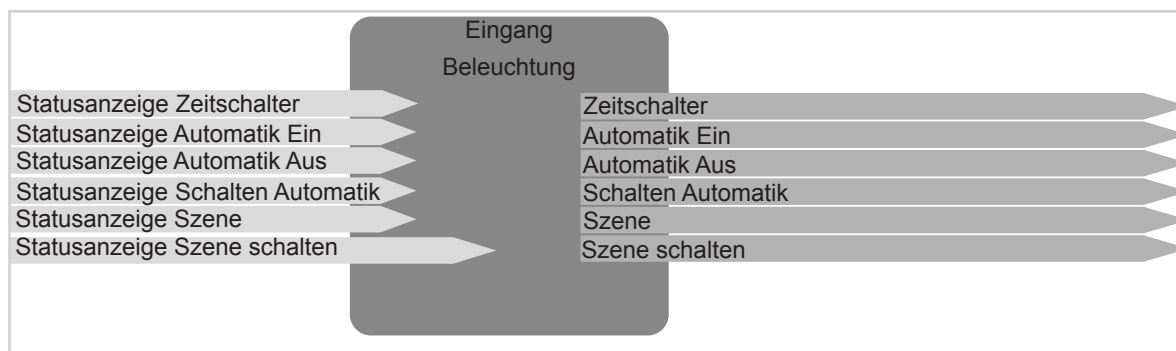
Bild 2: Ein-/Ausgangssignale Funktion Beleuchtung
