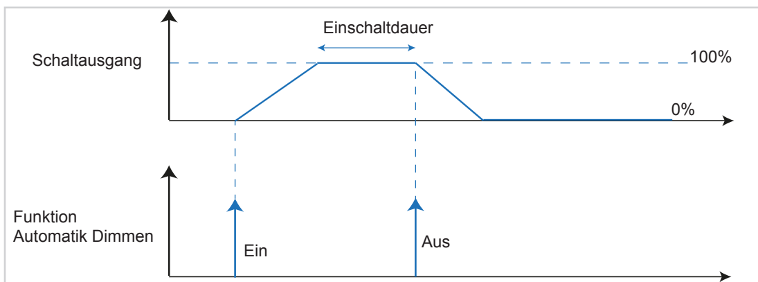
Bild 28: Signal-Zeit-Diagramm Automatik Dimmen
