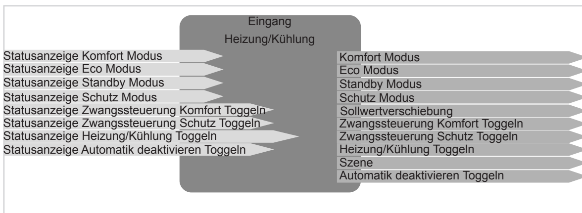
Bild 5: Ein-/Ausgangssignale Funktion Heizung/Kühlung
