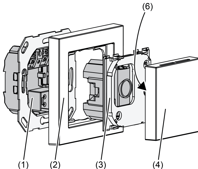
Bild 2: Gerätemontage
