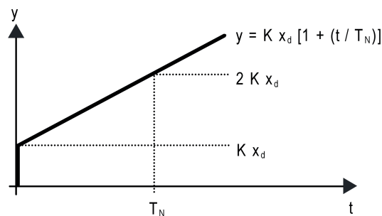
Bild 24: Funktion der Stellgröße einer PI-Regelung
