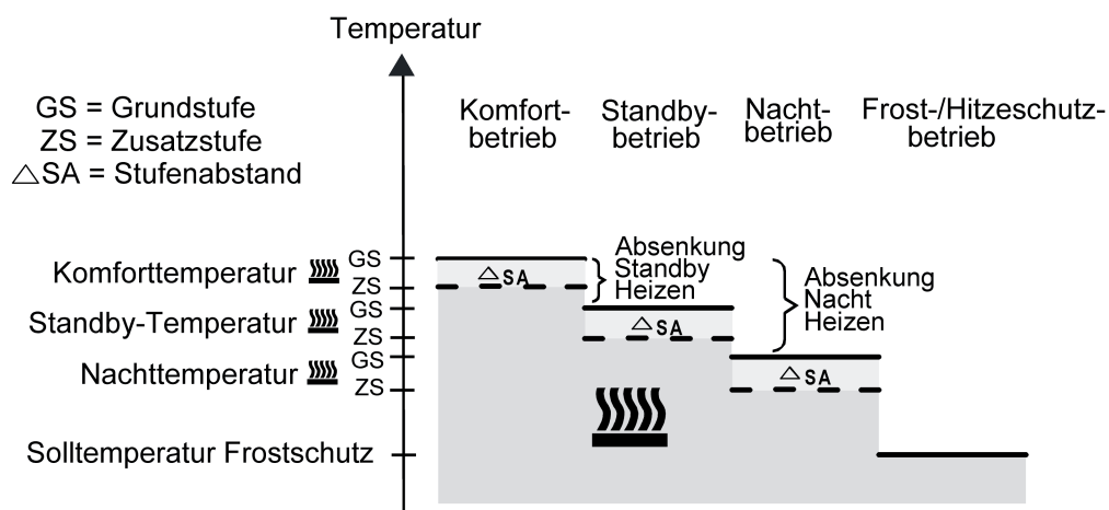
Bild 31: Solltemperaturen in der Betriebsart "Grund- und Zusatzheizen"
