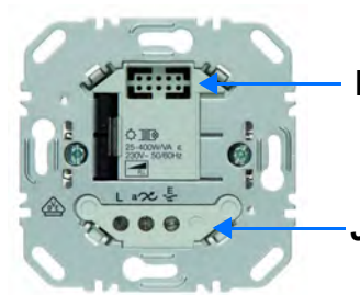
1 sortie variateur
