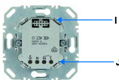
1 overdrachtsuitgang
