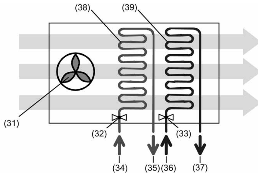
Bild 9: Das 4-Rohr-System
