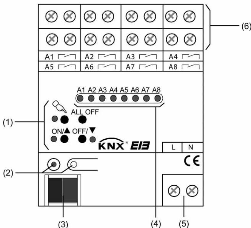
Bild 1: Geräteaufbau
