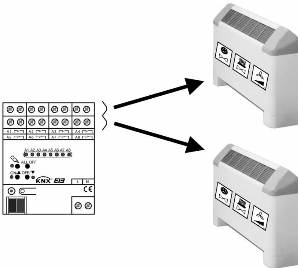
Bild 11: Der 2-Kanal-Betrieb
