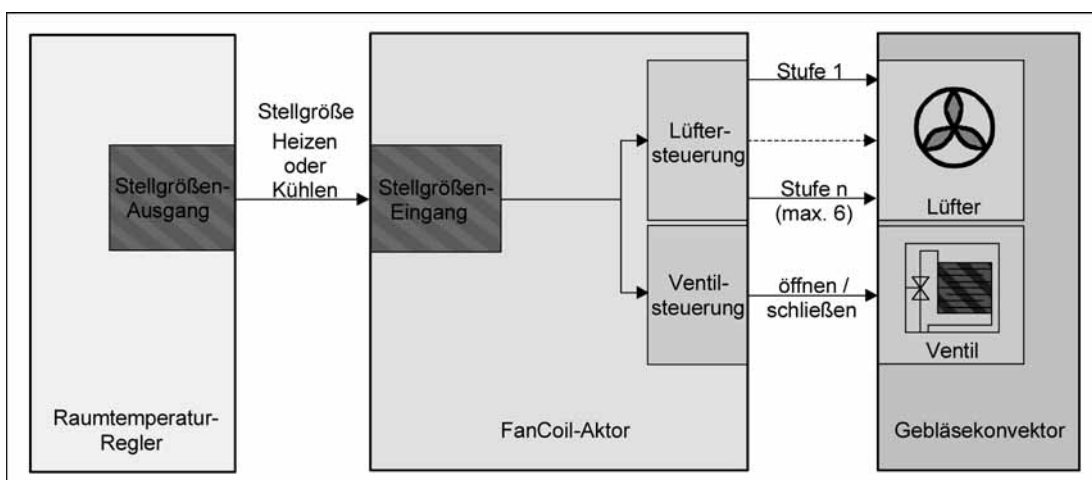
Bild 12: Funktionsschema "2-Rohr nur Heizen" und "2-Rohr nur Kühlen"
