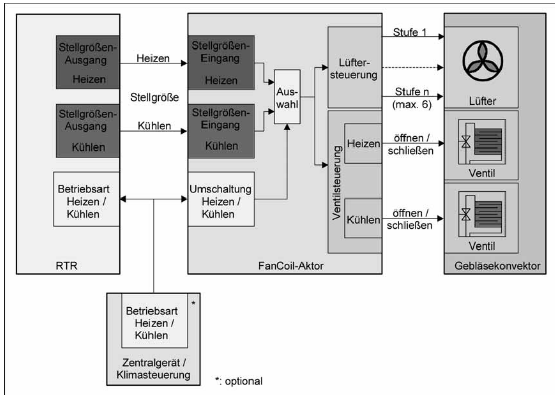
Bild 14: Funktionsschema "4-Rohr Heizen/Kühlen über Umschaltobjekt"
