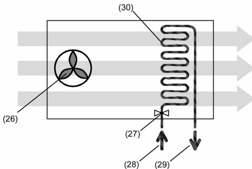
Bild 8: Das 2-Rohr-System
