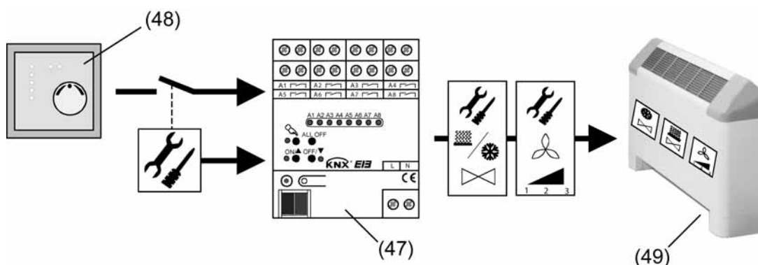
Bild 32: Prinzip der Sperrfunktion am Beispiel einer Wartungsverriegelung
