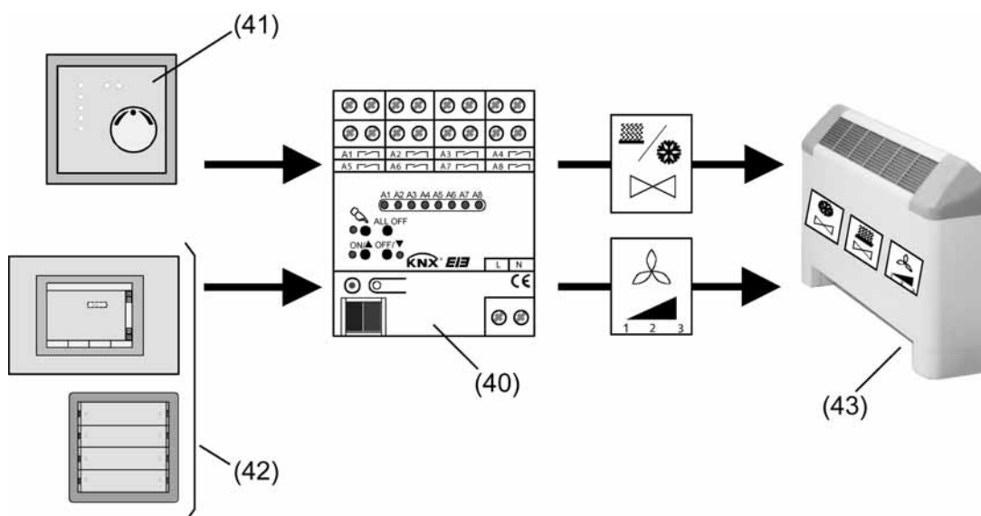
Bild 28: Prinzip der manuellen Lüftersteuerung
