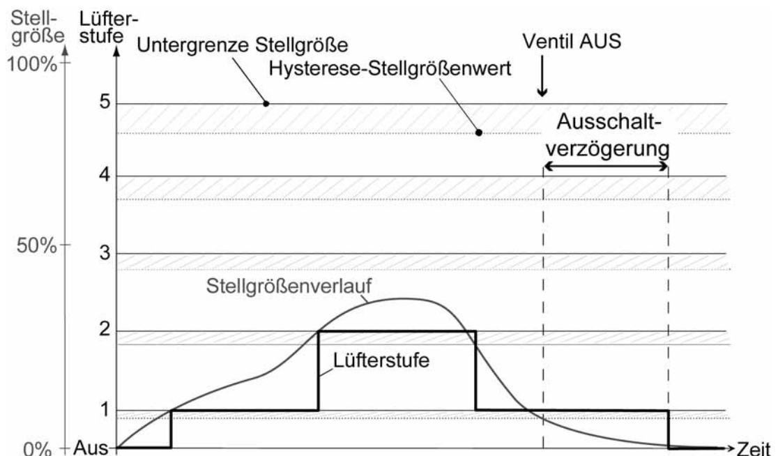
Bild 24: Vereinfachtes Stellgrößendiagramm zur Verdeutlichung einer Lüfterstufenumschaltung (aktive Lüfterstufe) unter Berücksichtigung einer Ausschaltverzögerung
