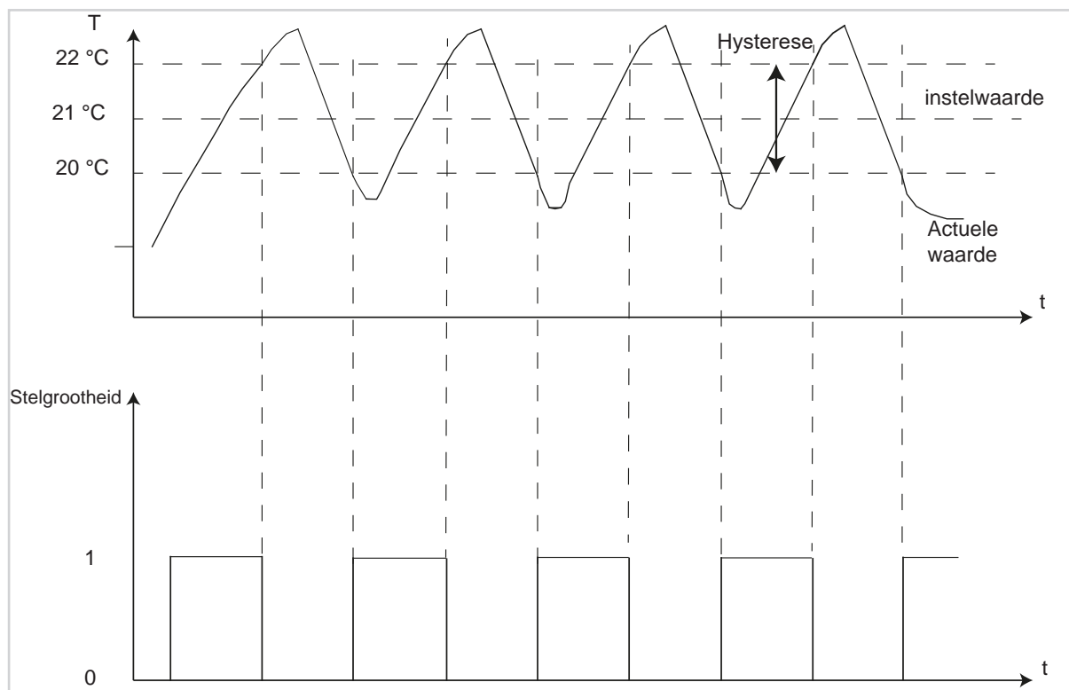
Afbeelding 18: 2-puntsregeling
