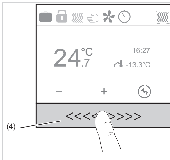
Afbeelding 4: slider-bediening
