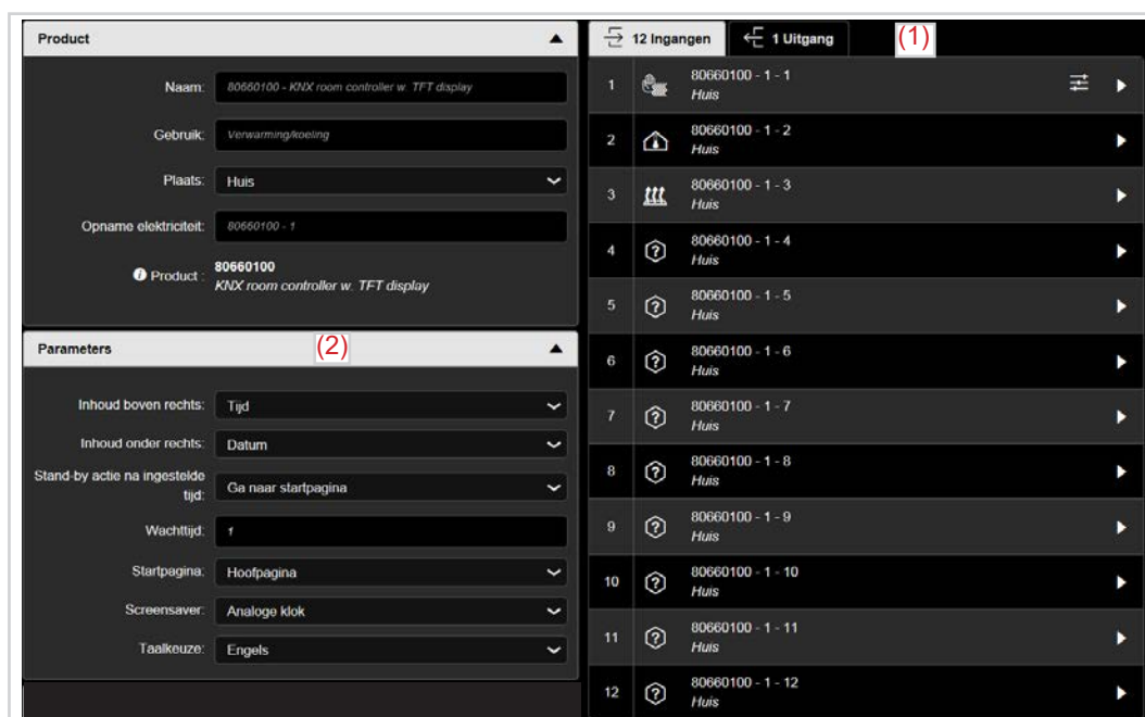
Afbeelding 10: Apparaat informatie
