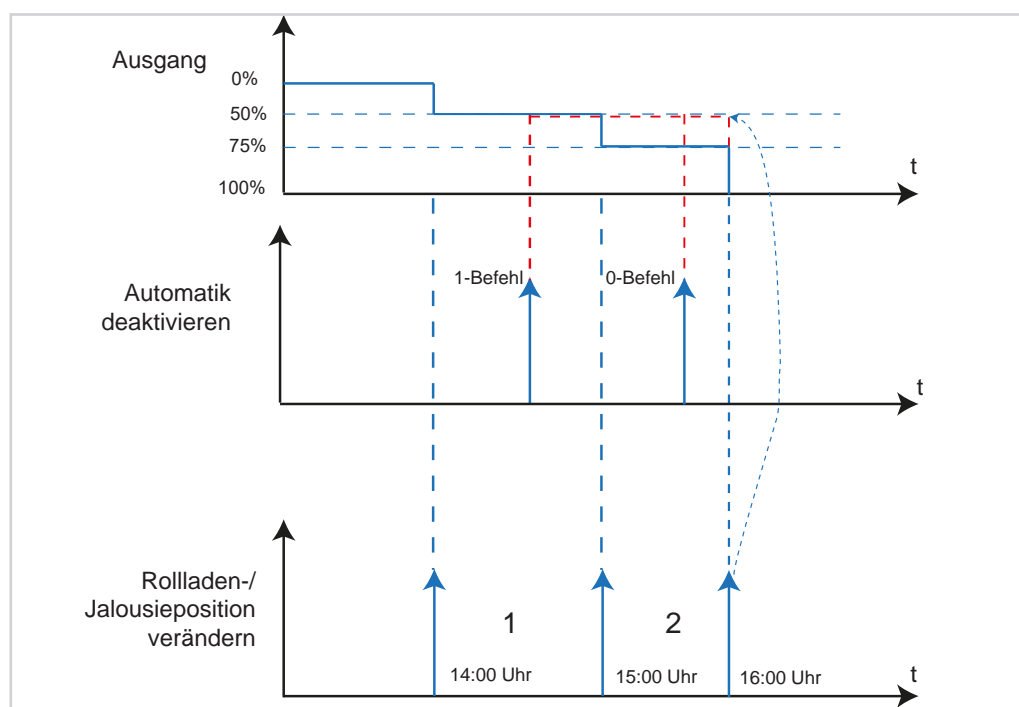
Bild 68: Signal-Zeit-Diagramm Automatik deaktivieren
