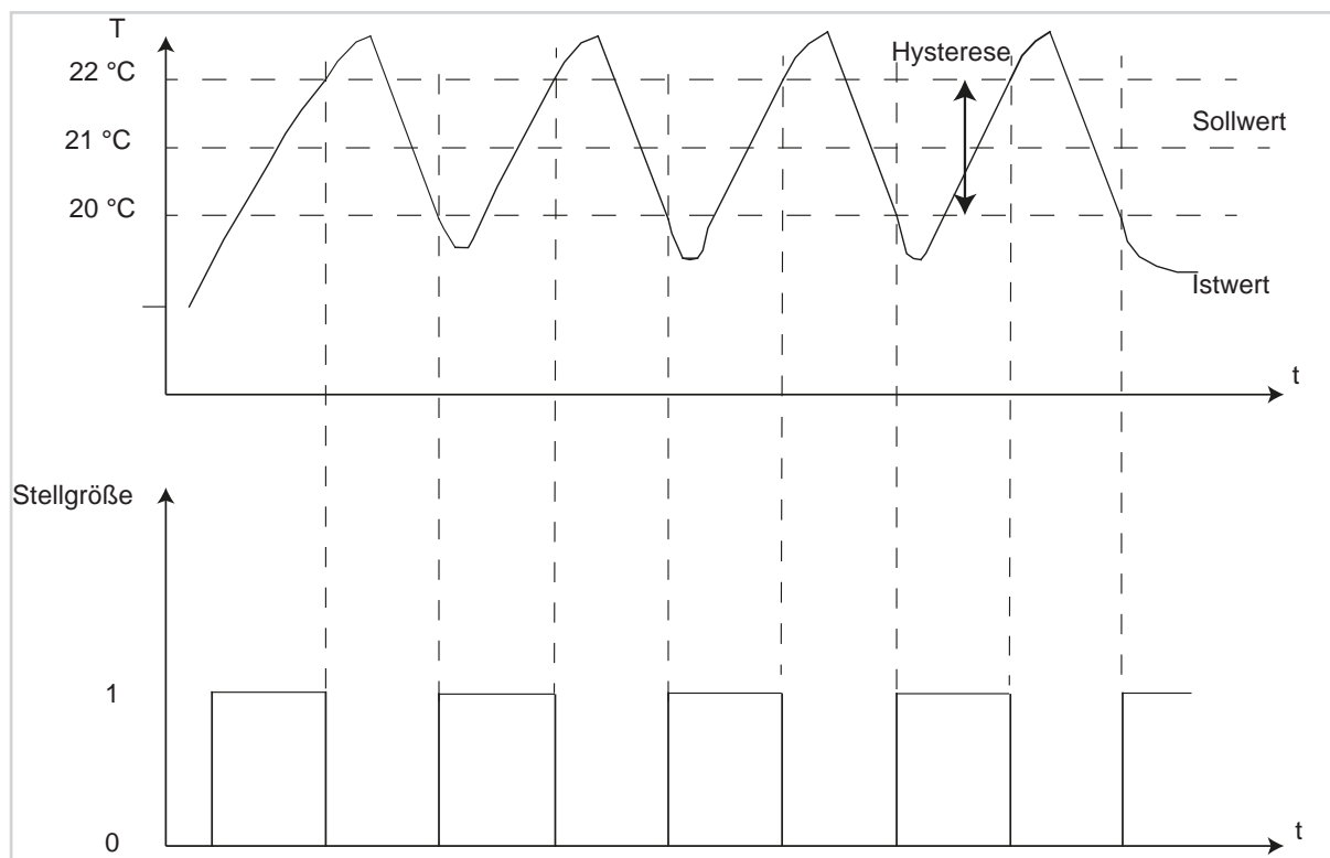
Bild 18: 2-Punkt-Regelung
