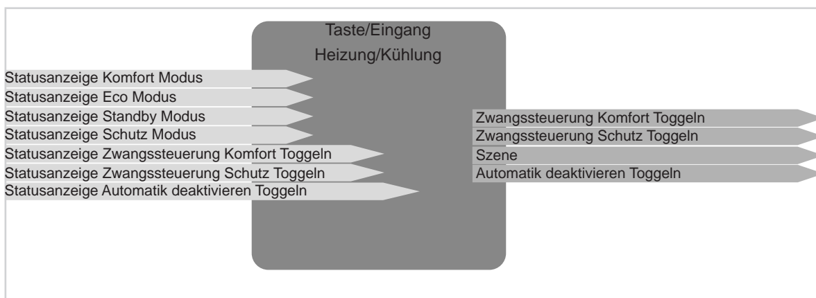
Bild 9: Ein-/Ausgangssignale Funktion Heizung/Kühlung
