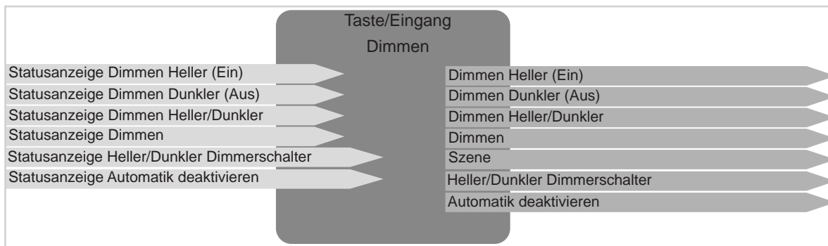
Bild 7: Ein-/Ausgangssignale Funktion Dimmen
