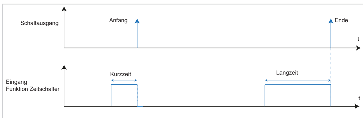
Bild 29: Signal-Zeit-Diagramm Zeitschalter
