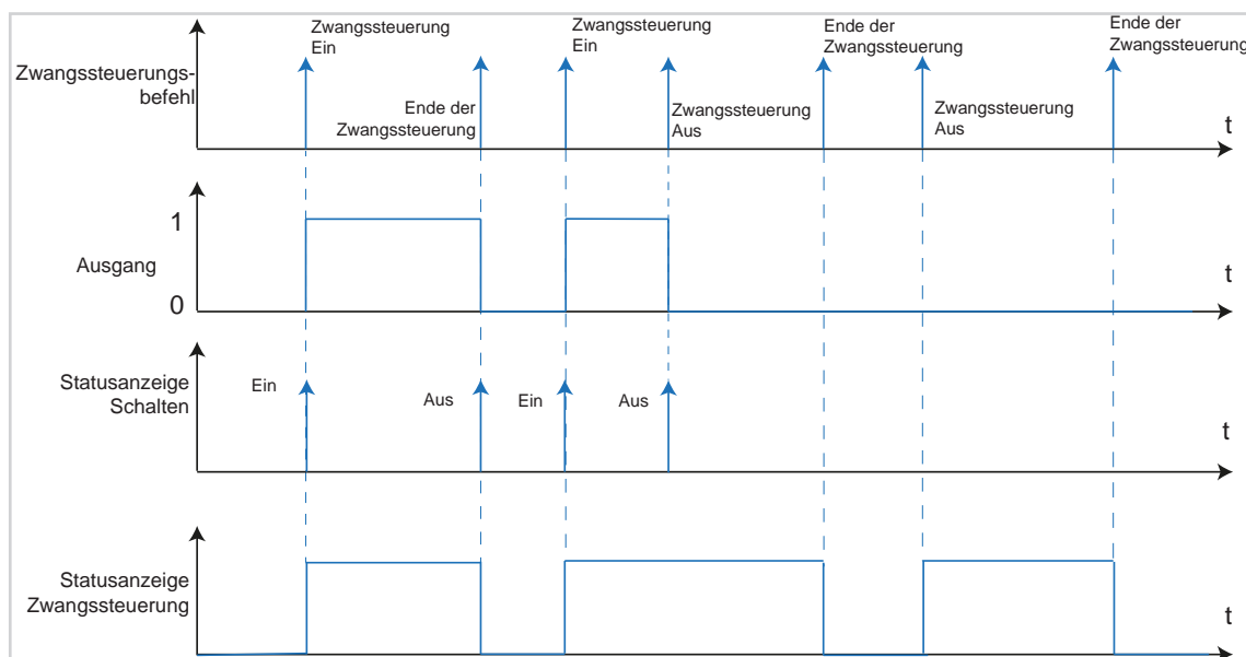
Bild 32: Signal-Zeit-Diagramm Zwangssteuerung
