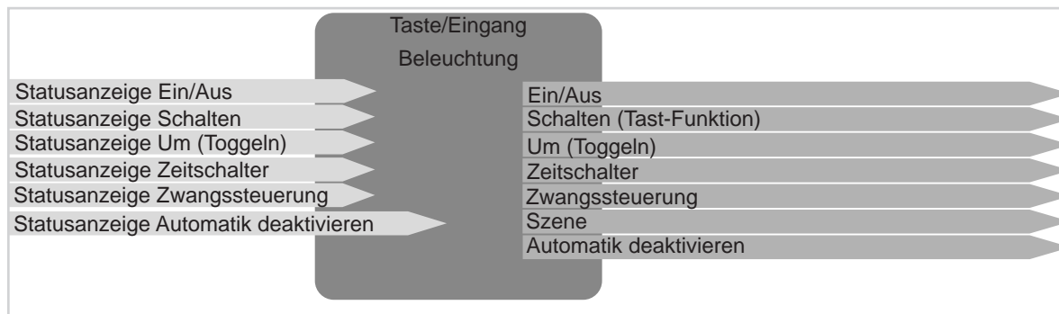
Bild 6: Ein-/Ausgangssignale Funktion Beleuchtung
