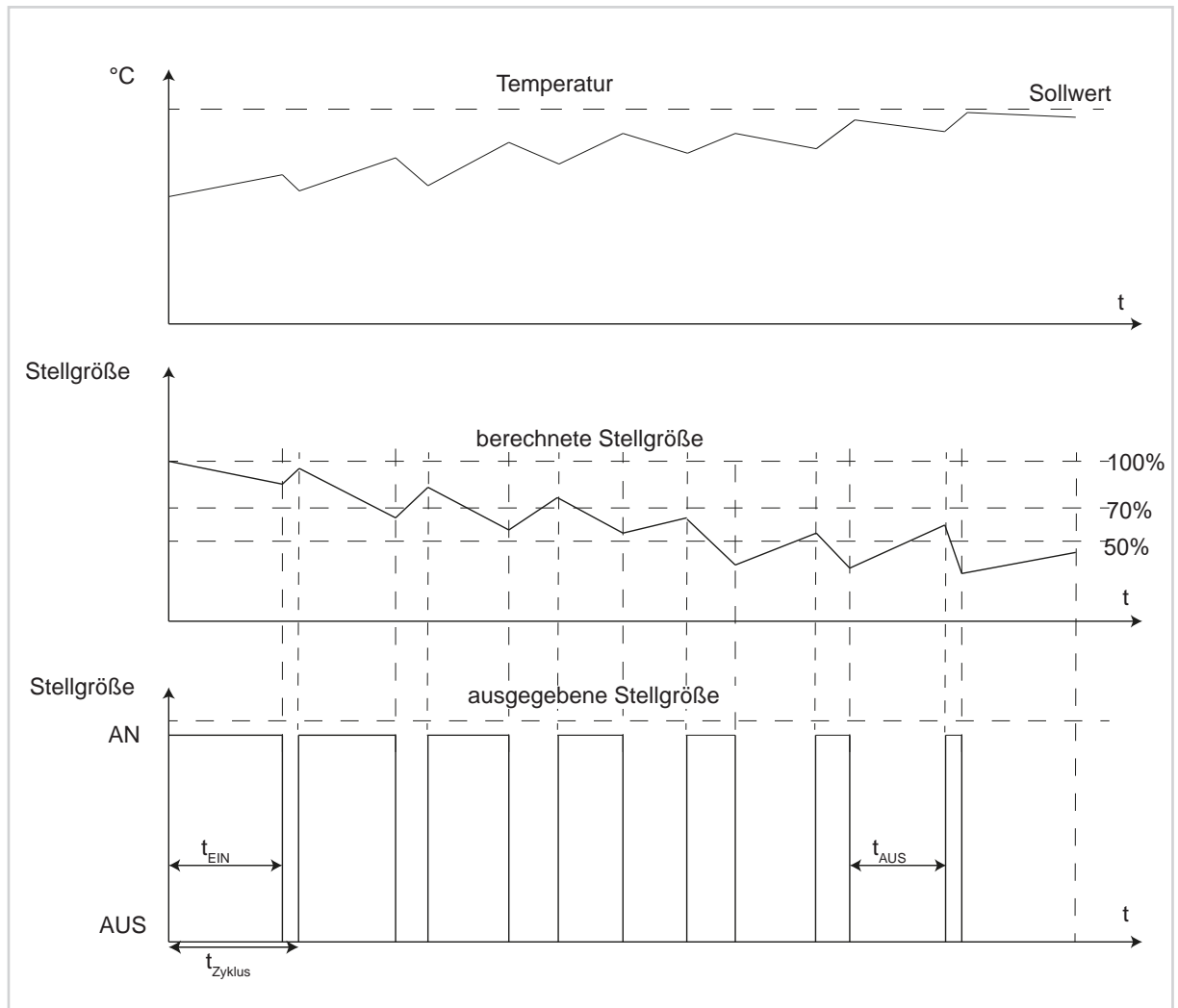
Bild 19: Schaltende PI-Regelung (PWM)
