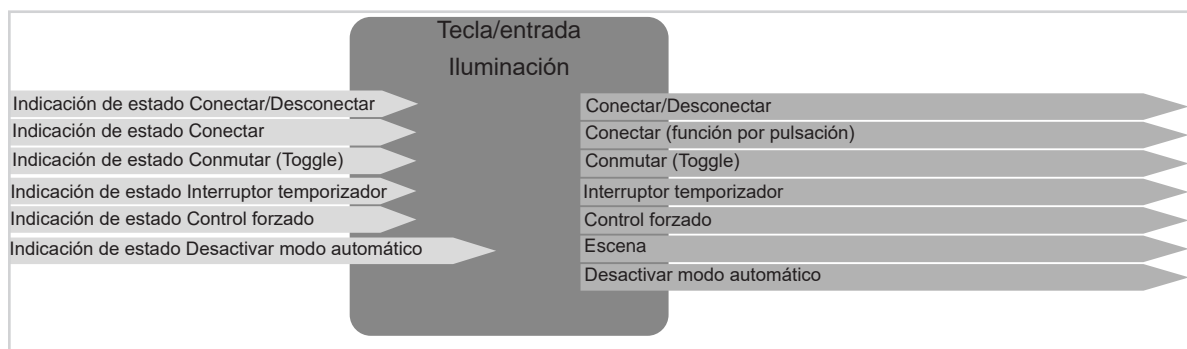
Figura 6: Señales de entrada/salida Función Iluminación
