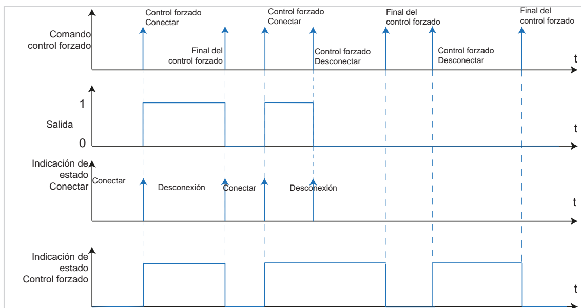
Figura 32: Gráfico señal-tiempo de control forzado
