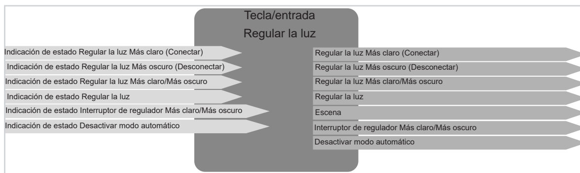
Figura 7: Señales de entrada/salida Función Regular la luz
