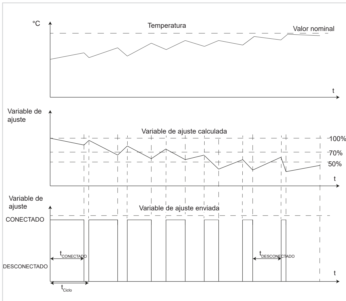
Figura 19: Regulación PI conmutada (PWM)
