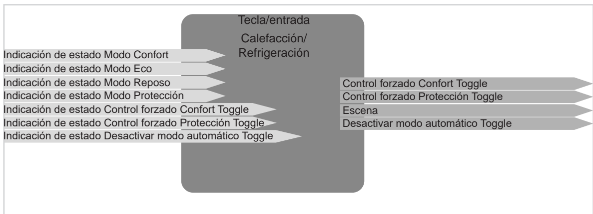
Figura 9: Señales de entrada/salida Función Calefacción/Refrigeración
