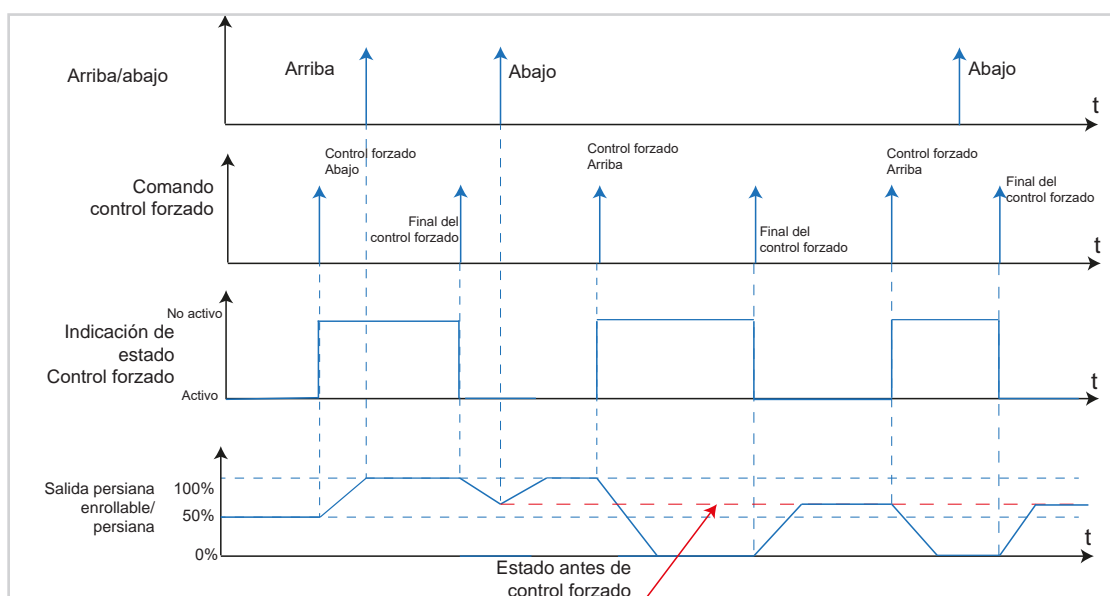
Figura 66: Gráfico señal-tiempo de Control forzado Persiana enrollable/Persiana
