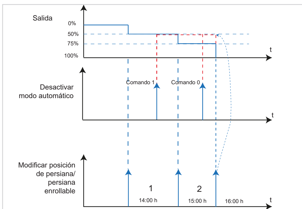
Figura 68: Gráfico señal-tiempo Desactivar modo automático
