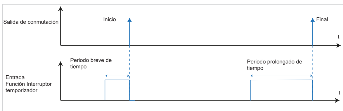
Figura 29: Gráfico señal-tiempo interruptor temporizador
