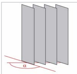
Figura 52: Ángulo de lamas en desplazamiento de apertura \alpha \approx 180^\circ
