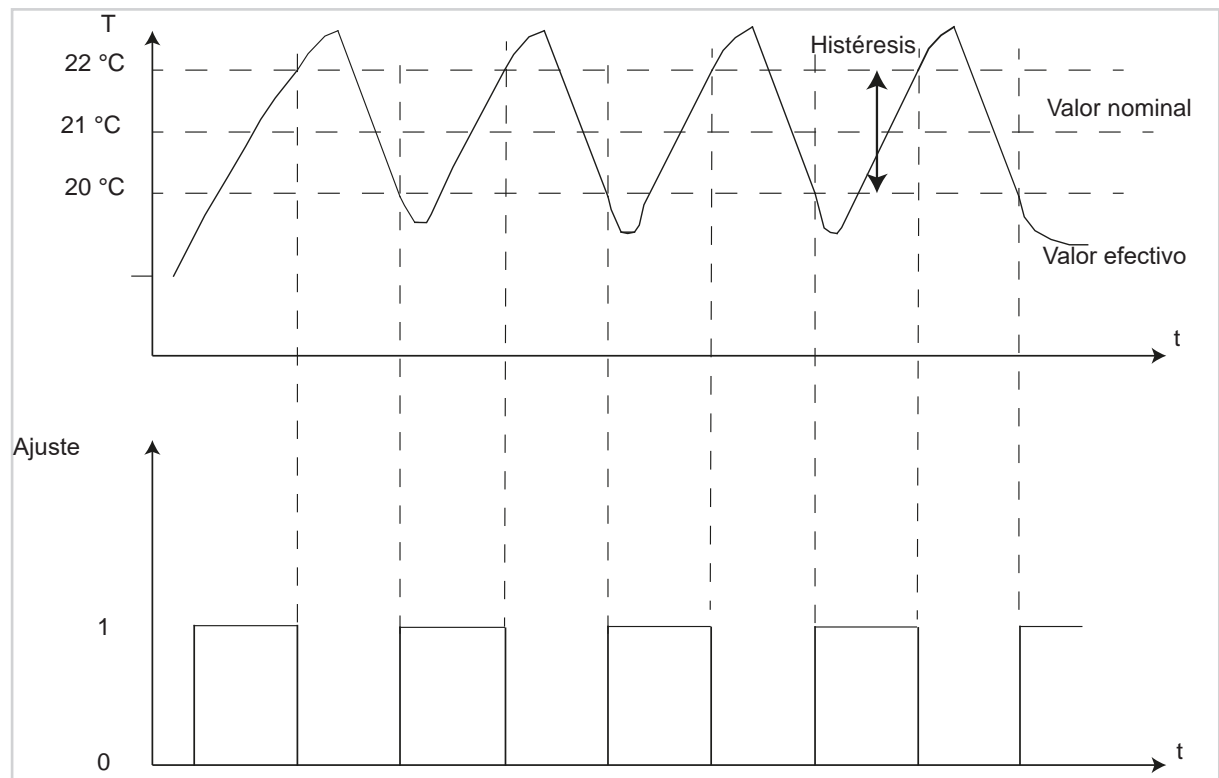
Figura 18: Regulación de 2 puntos
