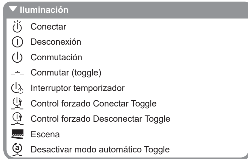
Figura 24: Vista general de la función Iluminación
