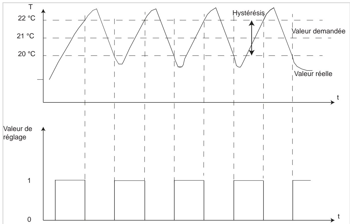
Image 18: Régulation à 2 points
