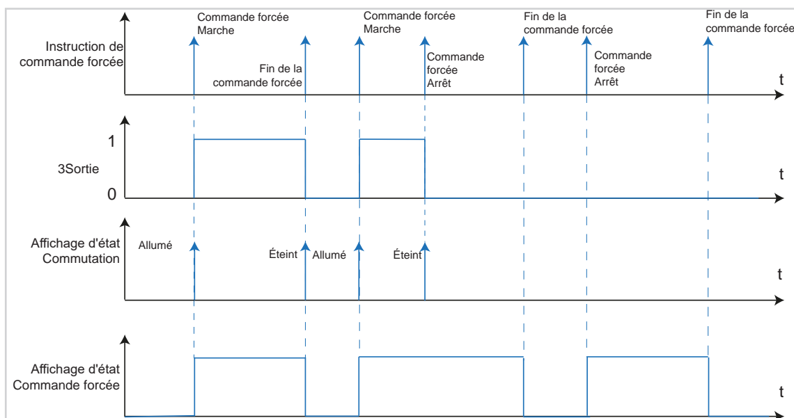
Image 32: Diagramme signal-temps Commande forcée
