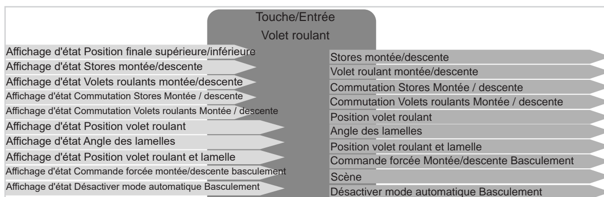
Image 8: Signaux d'entrée / de sortie Fonction Volet roulant
