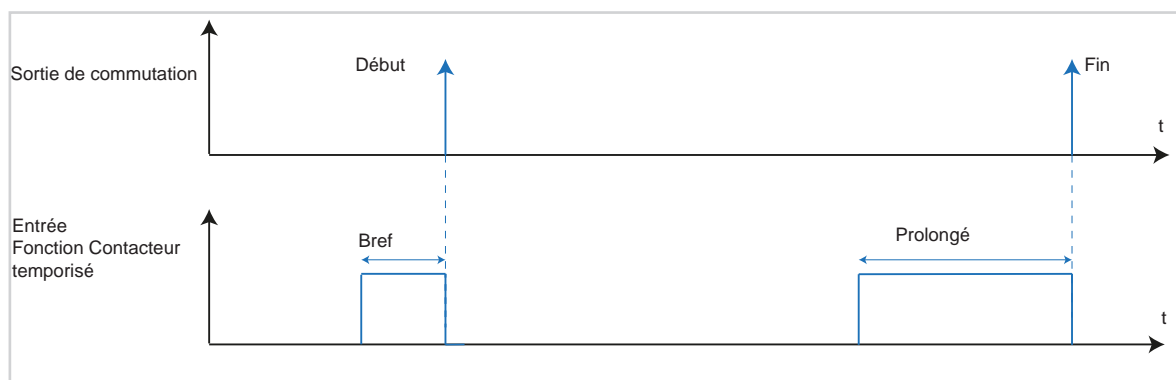
Image 29: Diagramme signal-temps Contacteur temporisé
