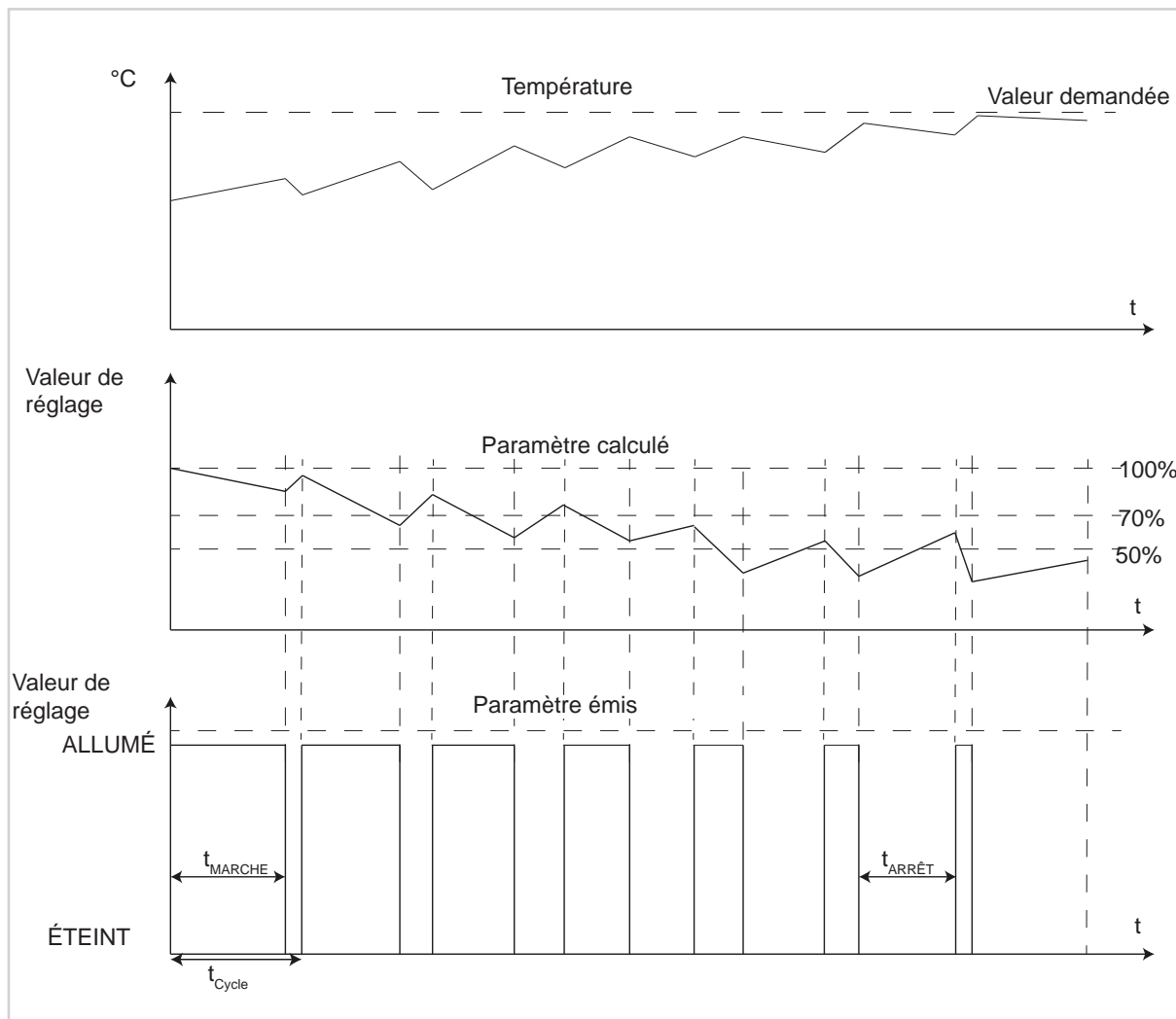
Image 19: Régulation PI tout-ou-rien (régulation MLI)
