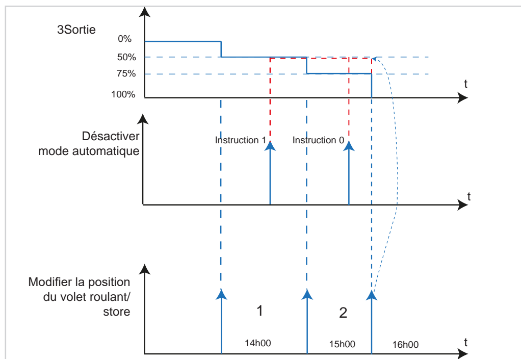
Image 68: Diagramme signal-temps Désactiver mode automatique
