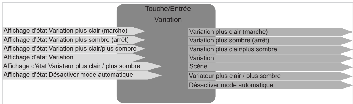
Image 7: Signaux d'entrée / de sortie Fonction Variation
