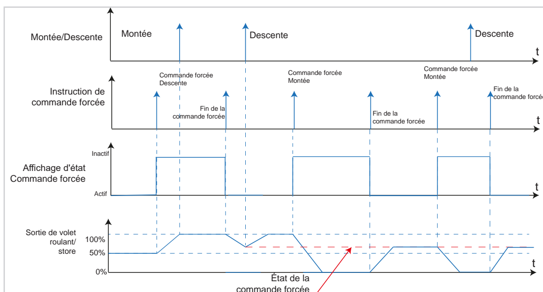
Image 66: Diagramme signal-temps Commande forcée Volet roulant/store
