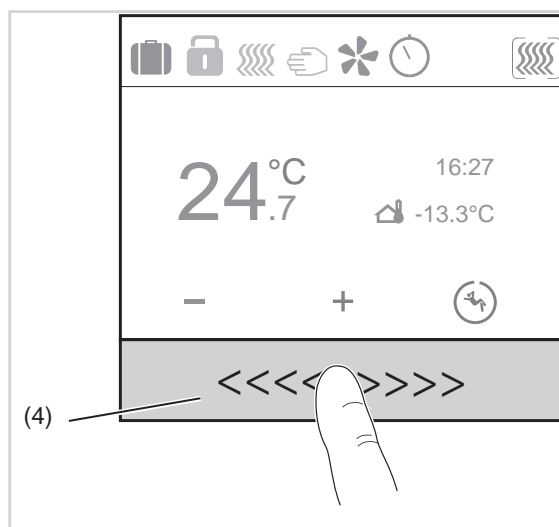
Image 4: Principe d'utilisation Fonctionnement curseur
