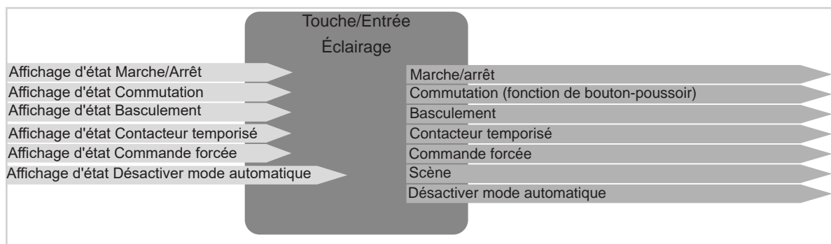
Image 6: Signaux d'entrée/de sortie Fonction Éclairage
