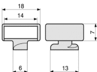
ZP2 Elément de fixation
