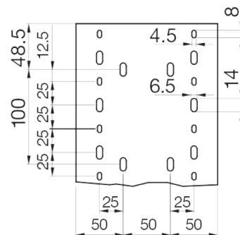
T1-N largeur 150 Perforation du socle
