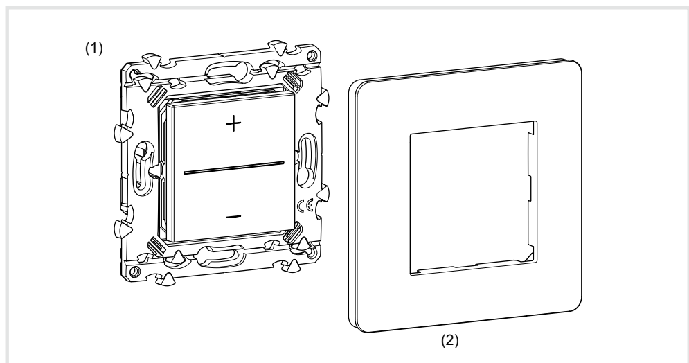
Image 1: Vue d'ensemble de l'appareillage
