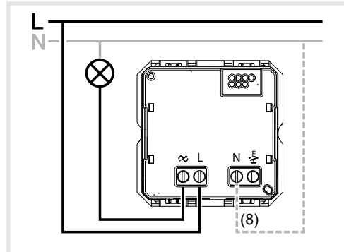
Image 3: Schéma de branchement (Circuit de base)
