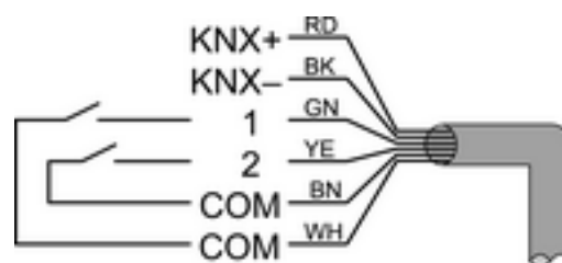
Afbeelding 2: Aansluitbezetting stuurkabel
