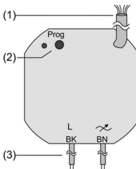
Afbeelding 1: Inbouwdimactor
