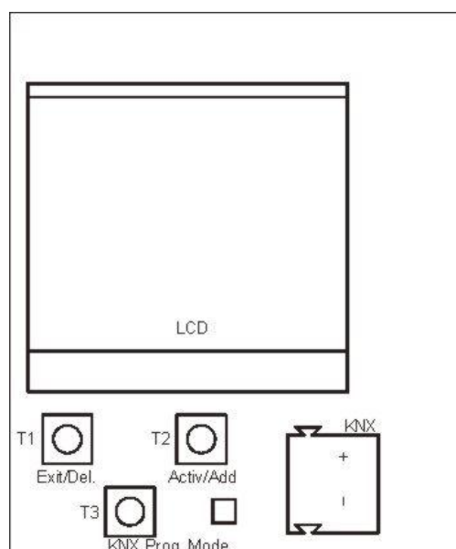
Abb. 2: Ansicht des geöffneten Gerätes
