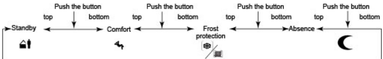
Image 28 : Modification de la valeur demandée du thermostat d'ambiance pour la fonction bascule
