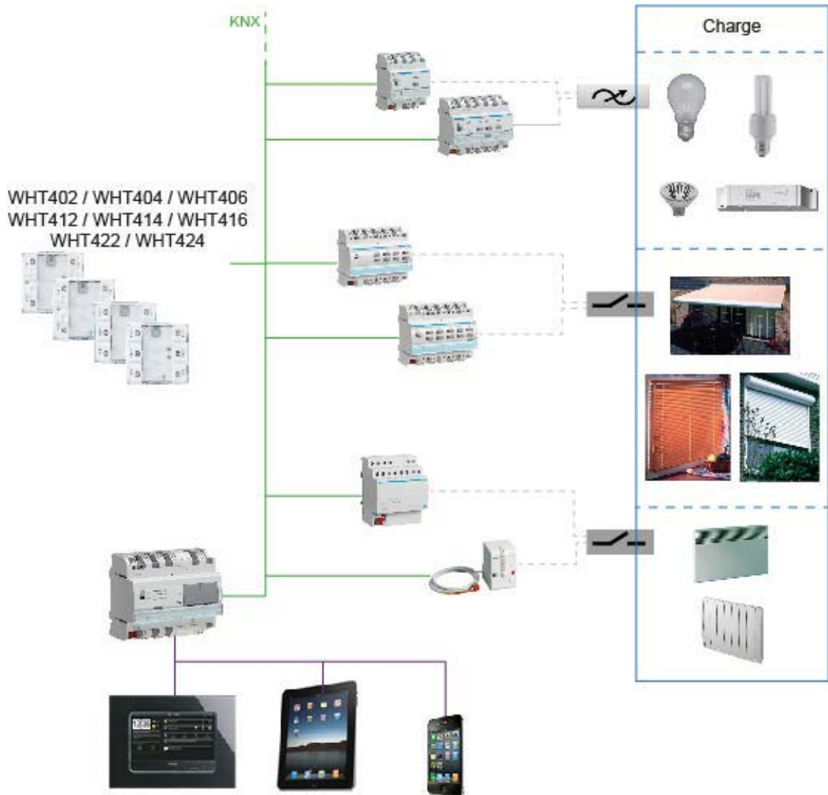
Image 1 : vue d'ensemble de l'appareillage
