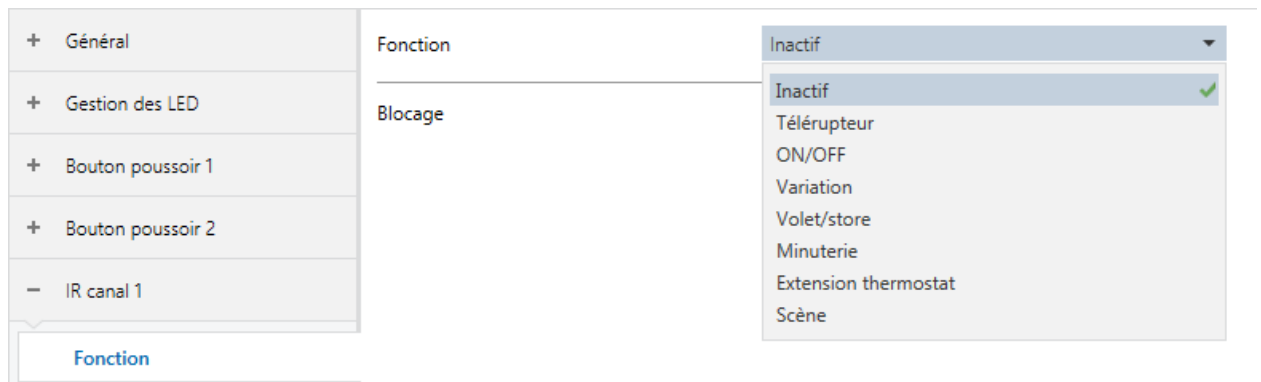
Image 42 : Paramètre de fonctionnement de l'interface IR
