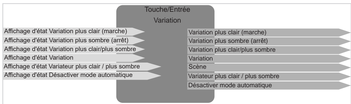
Image 7: Signaux d'entrée / de sortie Fonction Variation
