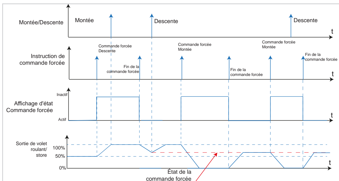
Image 66: Diagramme signal-temps Commande forcée Volet roulant/store
