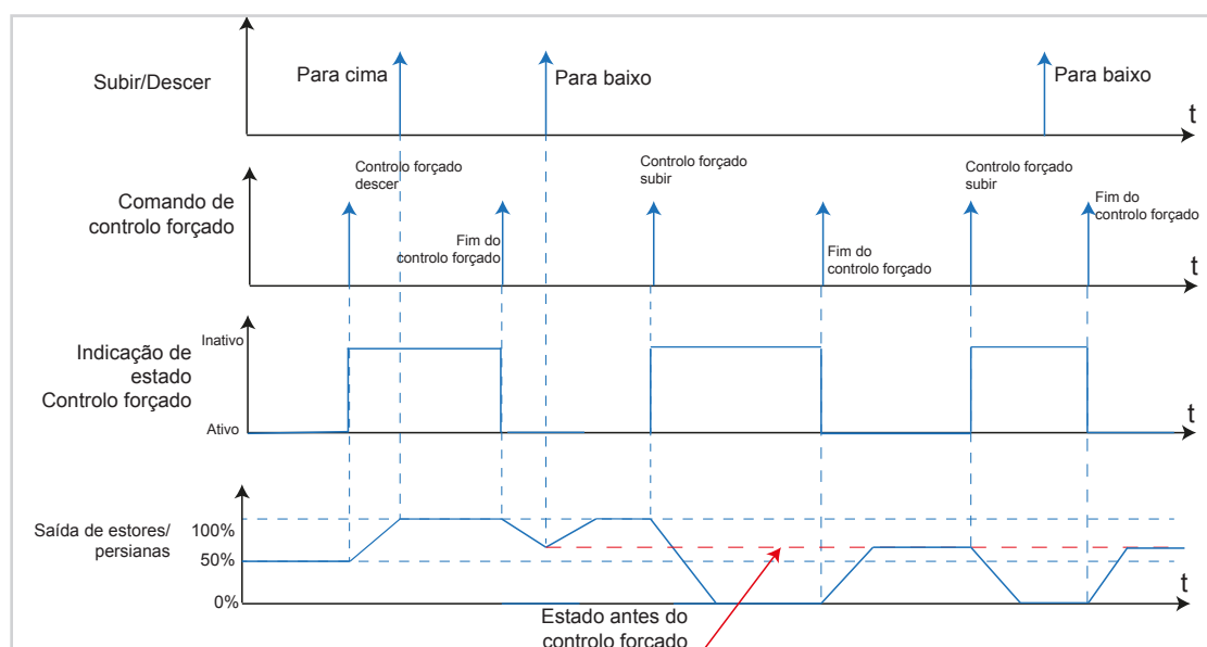
Figura 51: Diagrama de sinal e tempo Controlo forçado estore/persiana
