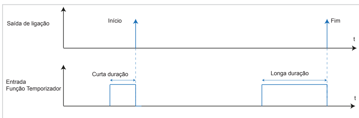
Figura 19: Diagrama de sinal e tempo Temporizador
