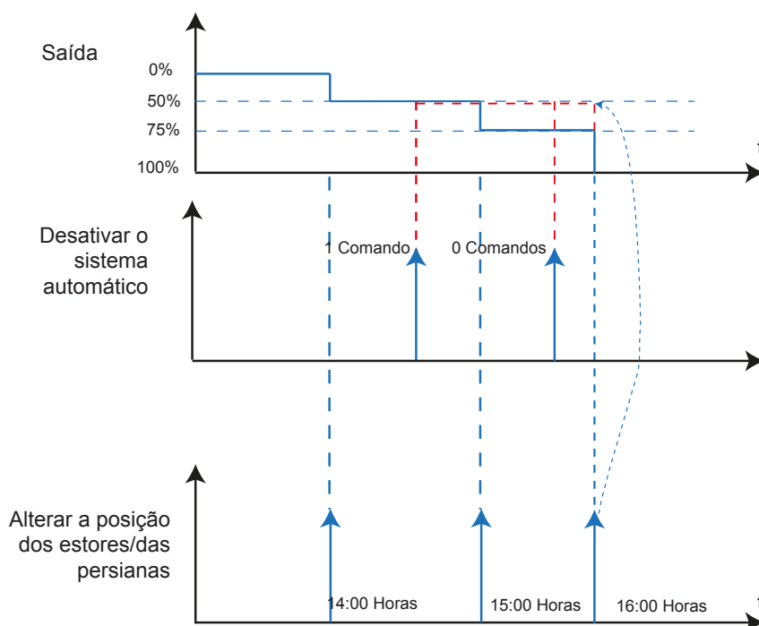
Figura 53: Diagrama de sinal e tempo Desativar o sistema automático
