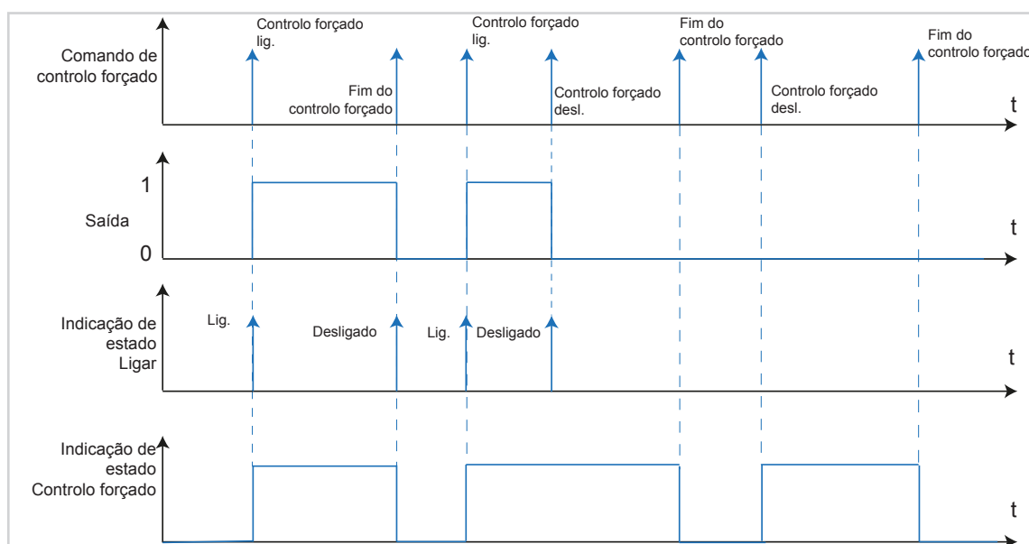
Figura 22: Diagrama de sinal e tempo Controlo forçado
