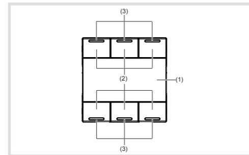
Figura 1: vista frontal pulsador 6 teclas con LED y retroiluminación, con o sin receptor IR
