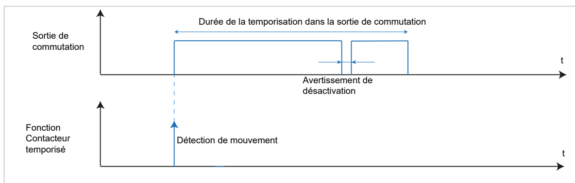
Image 11: Diagramme signal-temps Contacteur temporisé
