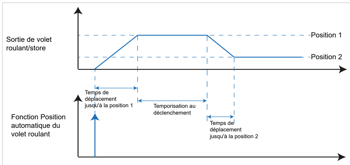
Image 53: Diagramme signal-temps Position automatique du volet roulant
