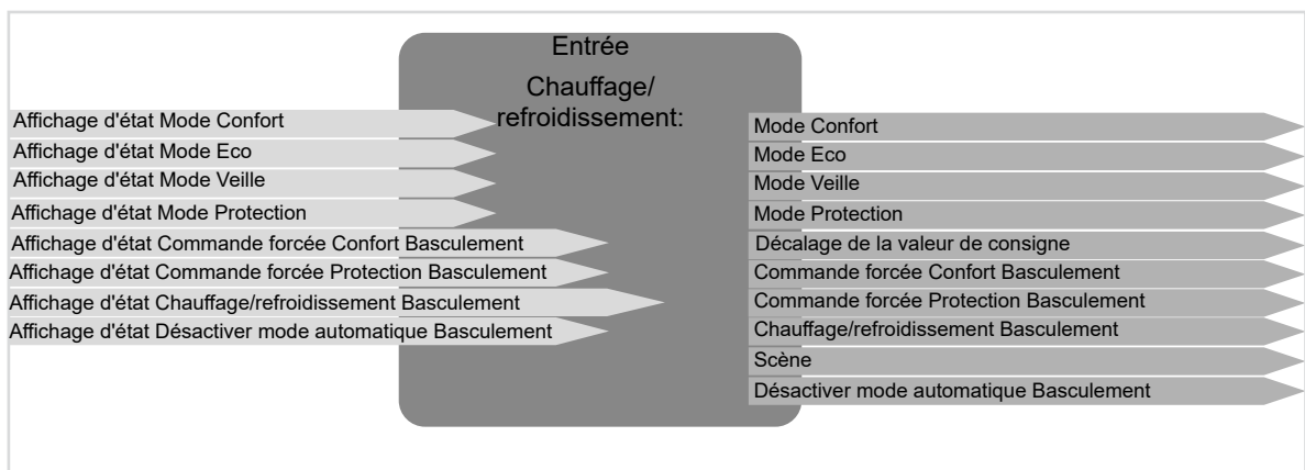
Image 5: Signaux d'entrée / de sortie Fonction Chauffage/refroidissement
