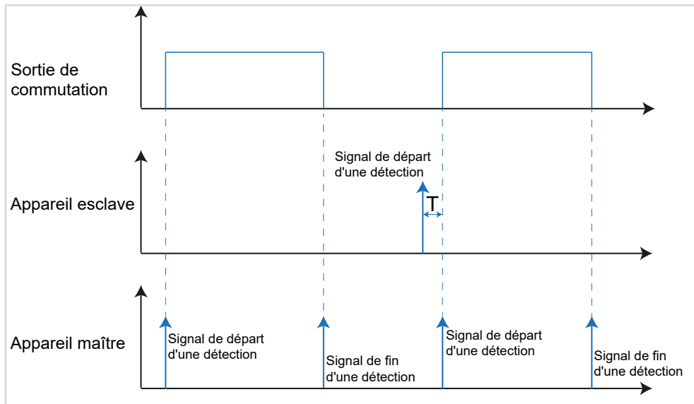
Image 70: Diagramme signal-temps Application maître - esclave
