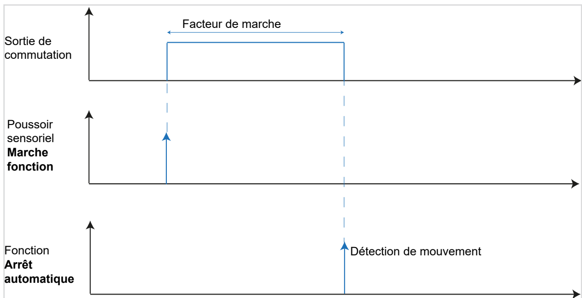
Image 15: Diagramme signal-temps Arrêt automatique
