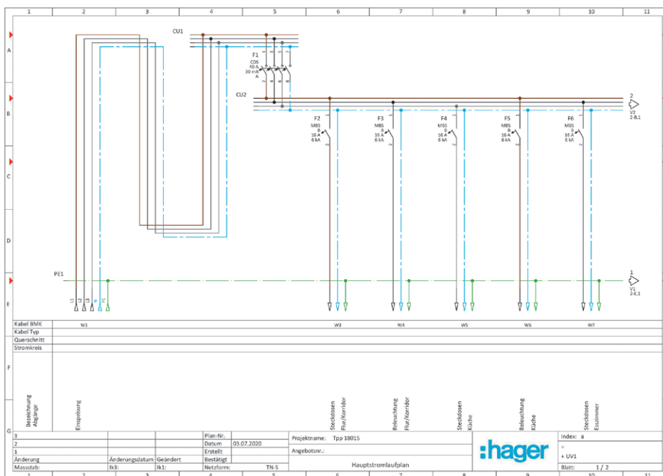
Abb. 4: Exemplarischer allpoliger Stromlaufplan
