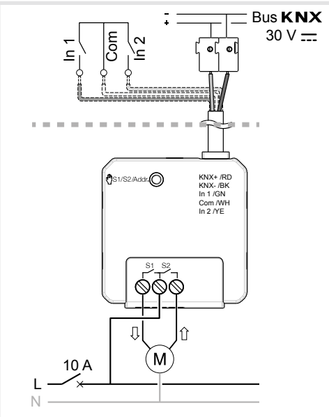
Figura 4: collegamento di motori
