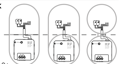
Bild 2: Installation mit getrenntem Anschlussraum
