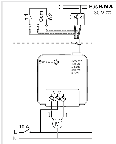
Bild 4: Anschluss von Motoren
