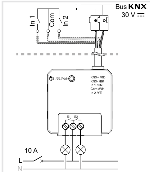
Figura 3: conexión de cargas de conmutación
