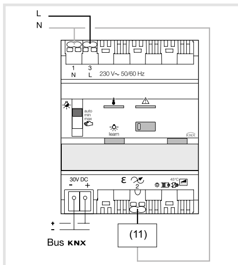
Figura 3: conexión del aparato
