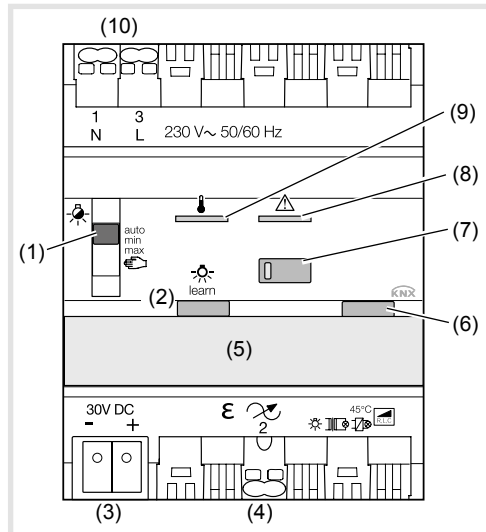
Figura 1: vista geral do aparelho
