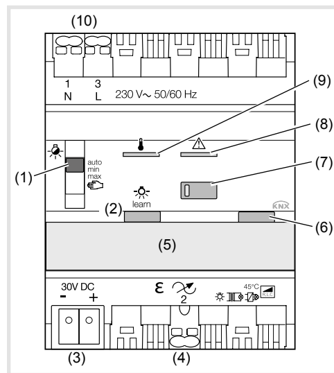
Figura 1: vista general del aparato
