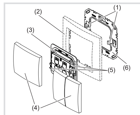
Bild 1: Geräteaufbau Wandsender
