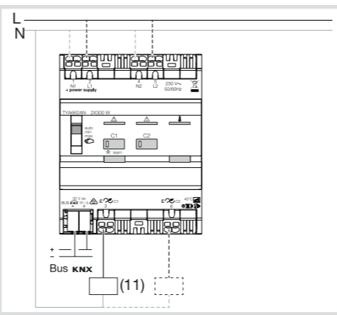
Image 3 : Installation monphasée
