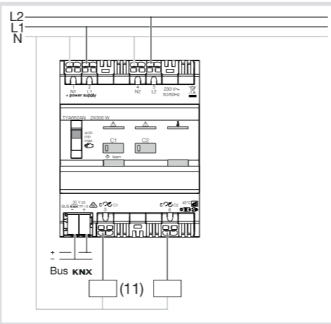
Image 4 : Installation triphasée
