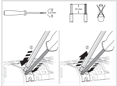
Afb. 2 : installatie/deinstallatie met steekklampen
