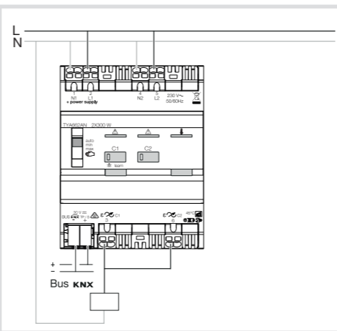
Image 5 : Combinaison de sortie (1+2)
