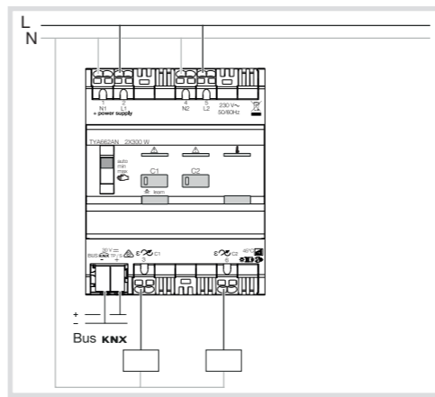
Image 6 : Combinaison de sortie (1)-(2)
