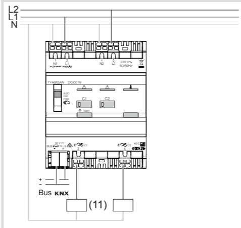
Afb. 4 : apparaat aansluiten meefasig
