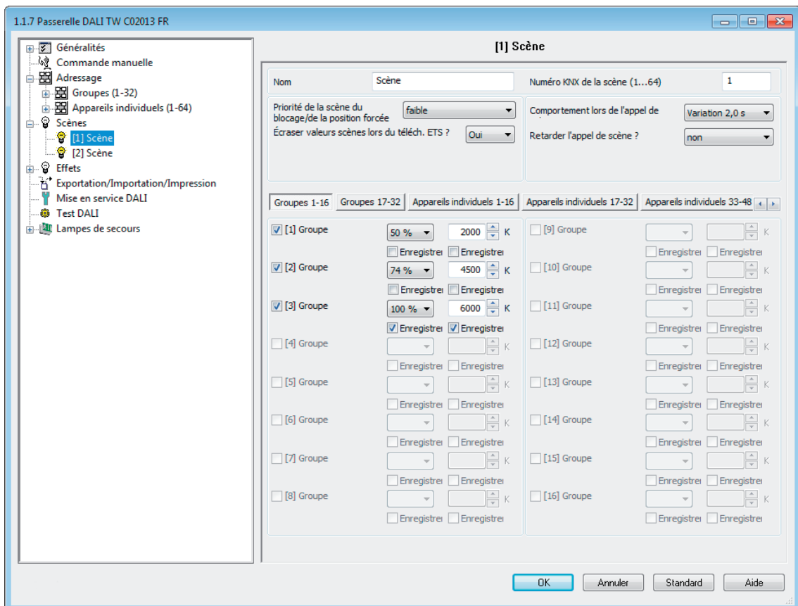
Figure 53: Page de configuration d'une scène à titre d'exemple avec deux scènes créées et trois groupes DALI
