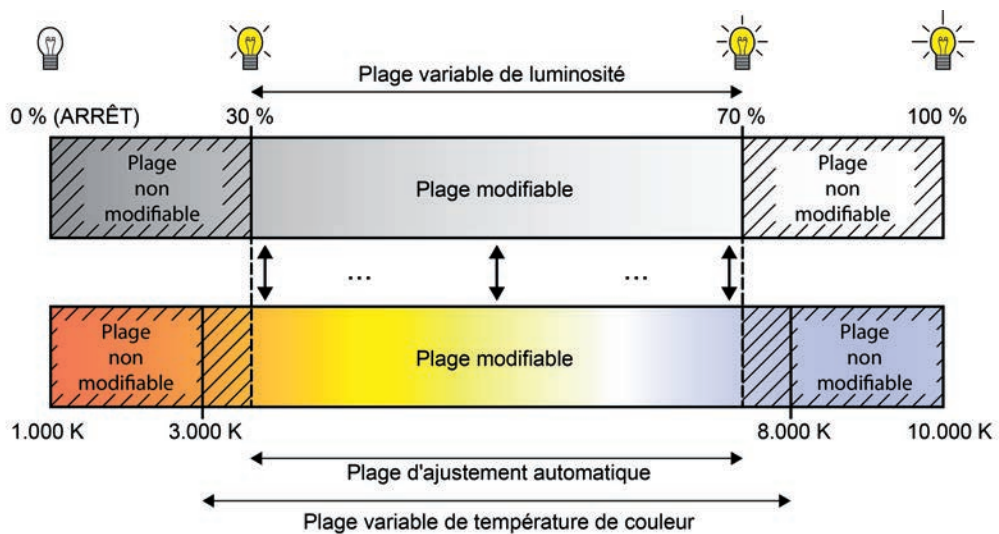
Figure 38: Adaptation automatique de la température de couleur à la luminosité réglée Exemple avec une plage de luminosité et de température de couleur restreinte
