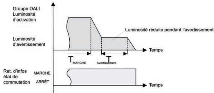
Figure 48: La fonction d'avertissement de la fonction cage d'escalier avec fonction ARRÊT progressif (exemple avec luminosité minimale = 0 %)
