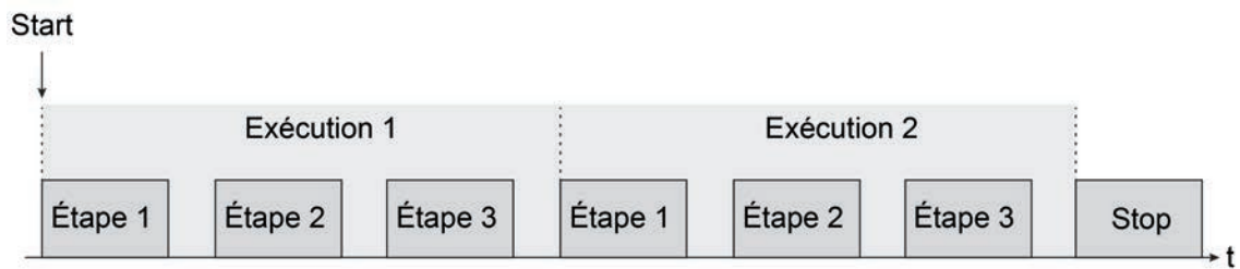
Figure 56: Exemple d'exécution d'un effet avec arrêt automatique (ici : 3 étapes d'effet, 2 exécutions)
