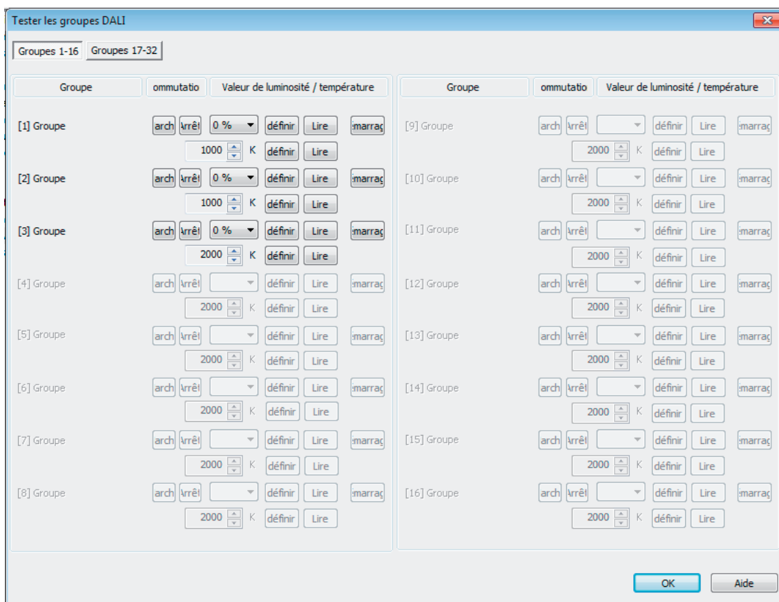
Figure 82: Environnement de test DALI orienté sur les groupes (exemple avec trois groupes créés)
