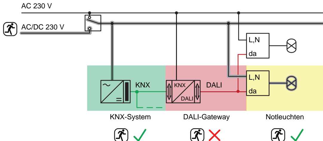
Bild 17: Beispiel einer Zentralversorgung - DALI-Betriebsgeräte und KNX-System in die Notstromversorgung eingebunden
