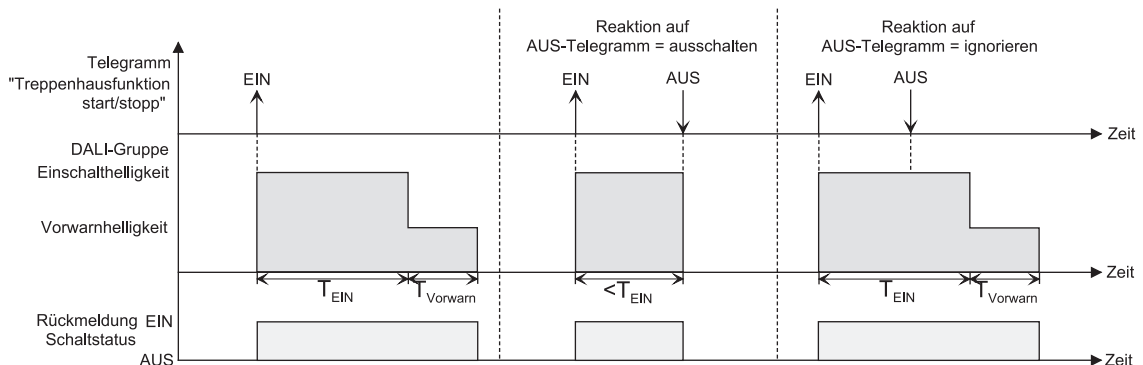
Bild 45: Ausschaltverhalten der Treppenhausfunktion ohne Soft-Funktionen
