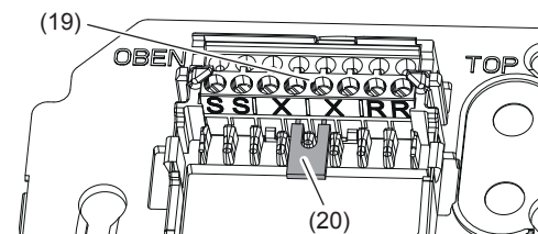
Bild 8: Anschluss-Klemmblock
