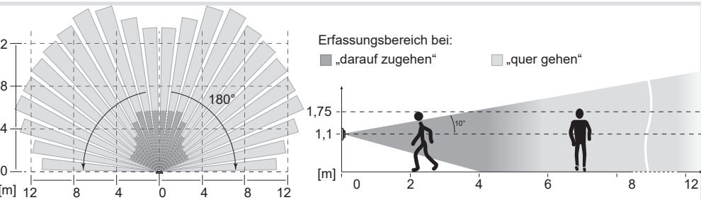
Bild 4a: Erfassungsbereich des Bewegungsmelders Montagehöhe 1,1 m
