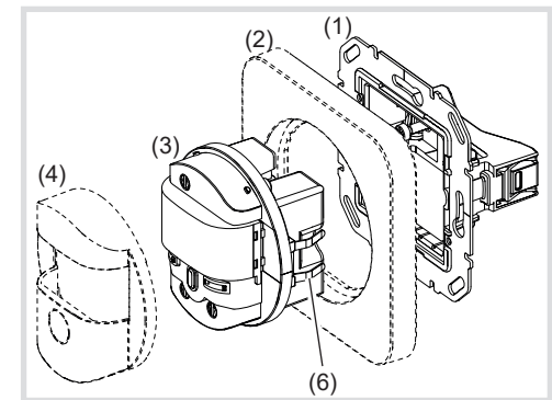
Bild 1b: Geräteaufbau R.1/R.3
