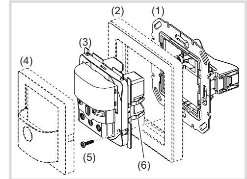
Bild 1a: Geräteaufbau
