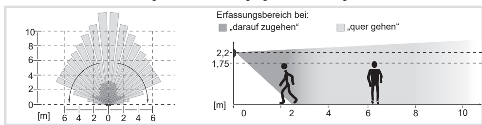
Bild 4b: Erfassungsbereich des Bewegungsmelders Montagehöhe 2,2 m
