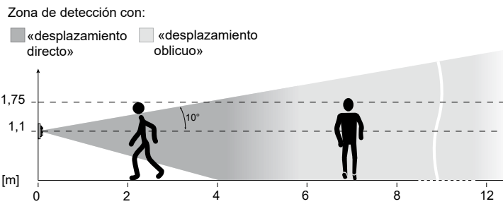
Figura 6: Zona de detección del detector de movimiento, altura de montaje de 1,1 m
