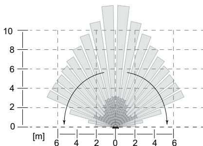
Figura 7: Zona de detección del detector de movimiento, altura de montaje de 2,2 m
