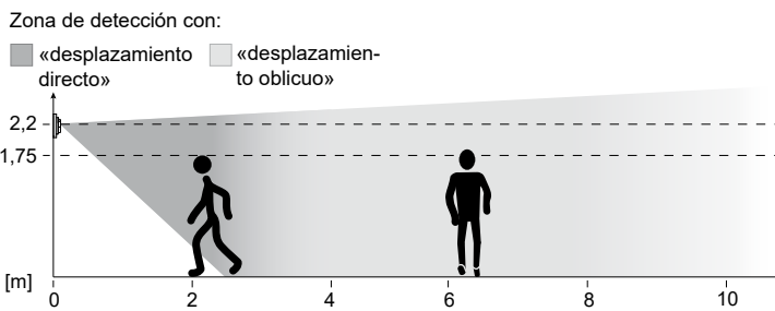
Figura 7: Zona de detección del detector de movimiento, altura de montaje de 2,2 m
