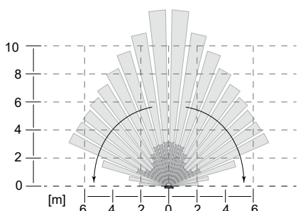
Figura 7: Área de detecção do detetor de movimento altura de montagem 2,2 m
