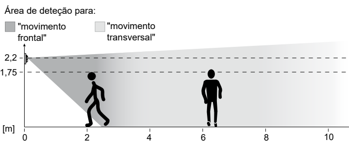
Figura 7: Área de detecção do detetor de movimento altura de montagem 2,2 m
