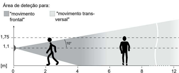
Figura 6: Área de detecção do detetor de movimento altura de montagem 1,1 m
