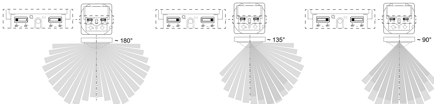
Figura 8: Regulação do ângulo de detecção
