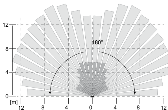
Figura 6: Área de detecção do detetor de movimento altura de montagem 1,1 m
