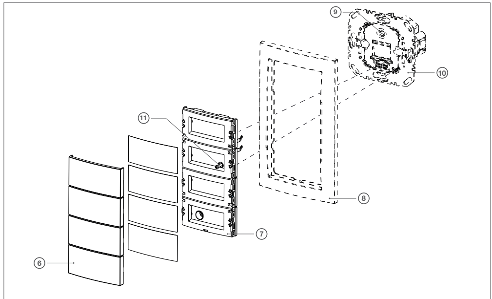
Resim 3: Cihazın monte edilmesi
