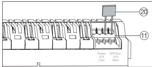
Abbildung 7: Anschluss des Abschlusswiderstands
