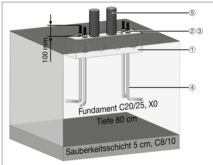
Abb. 17: Einbausockel einbetonieren
