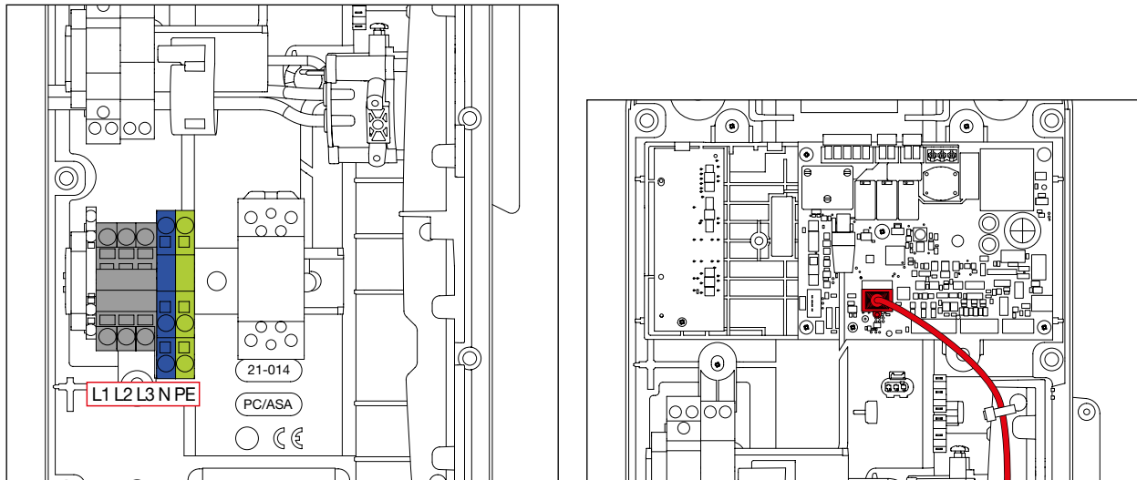
Abb. 25: Übersicht der Ethernet- und AC-Anschlüsse in der Ladestation
