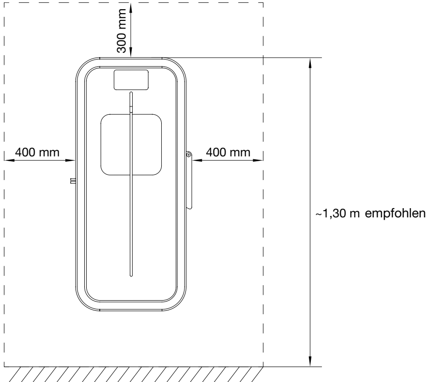
Abb. 4: Mindestabstände zu den Seiten und nach oben
