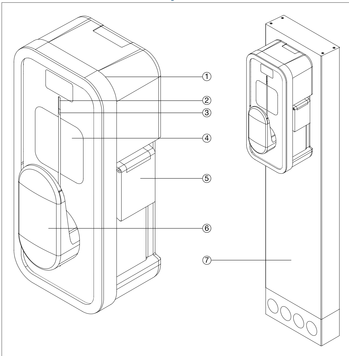
Abb. 2: Außenansicht der Ladestation witty solar
