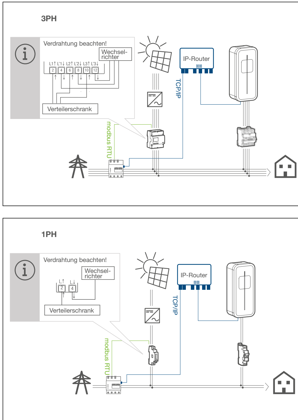
Abb. 24: Installation mit Photovoltaikanlage
