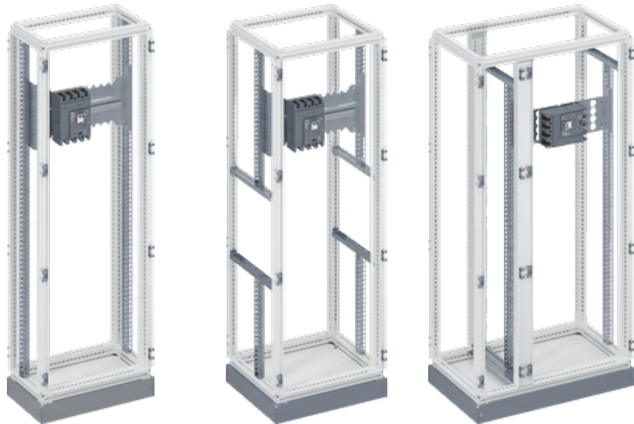
Exemple de configuration des montants fonctionnels
