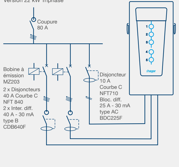
Coffret de protection Version 22 kW Triphasé
