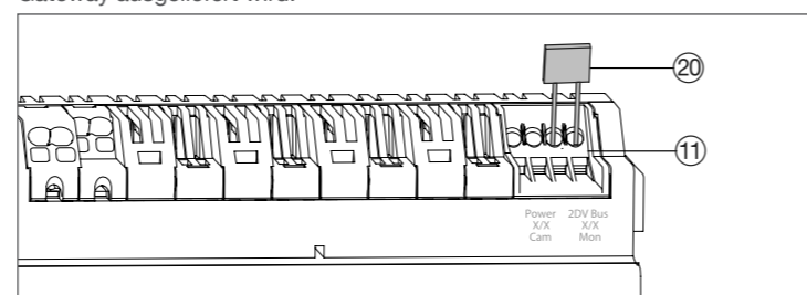
Abbildung 7: Anschluss des Abschlusswiderstands
