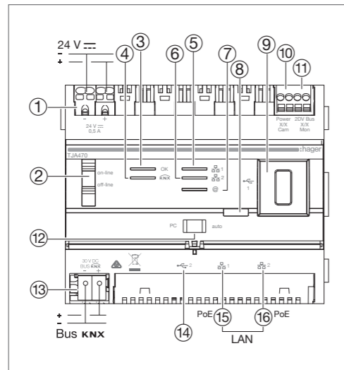
Bild 1: Aufbau des Geräts
