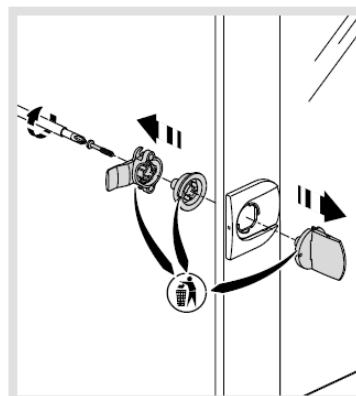
Schéma de montage / démontage
